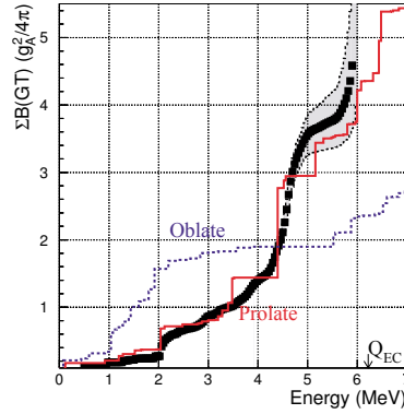
Figure E.1: Comparación de la distribución experimental de B(GT) acumulada con predicciones teóricas [Sar01] para deformación oblada (línea azul) y prolada (línea roja) del estado fundamental de ^{76}\text{Sr} [Nd04b]. La distribución experimental de B(GT) acumulada es similar a la predicción para el caso prolado lo cual sugiere este tipo de deformación para el estado fundamental del núcleo N=Z ^{76}\text{Sr} .
