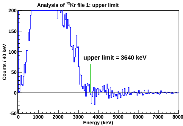
Figure E.4: Espectro correspondiente a la medida del fichero 1 de la desintegración de ^{72}\text{Kr} una vez han sido ya sustraídas las contaminaciones, a modo de ejemplo. Se indica el límite superior en energía que es elegido en el análisis para el espectro energético. La razón principal para esta elección es que a partir de esta energía el espectro muestra oscilaciones alrededor de número de cuentas cero alternando entre canales con estadística negativa y positiva.
