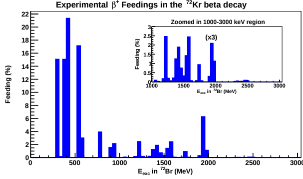
Figure E.5: Distribución de alimentación \beta^+ mostrado en la ventana energética hasta el valor Q_{\beta^+}=4105 keV obtenida a partir del análisis del espectro TAS, con condición de coincidencia con el detector \beta , imponiendo un límite superior en el análisis a una energía de 3640 keV en la medida del fichero 1 para la desintegración de ^{72}\text{Kr} . Las alimentaciones son encontradas hasta una energía de excitación de 2620 keV por las razones expuestas en el texto. El canal del gráfico insertado que está etiquetado con "(x3)" tiene su estadística reducida un factor 3 para que pudiese ser visto por completo en el gráfico.
