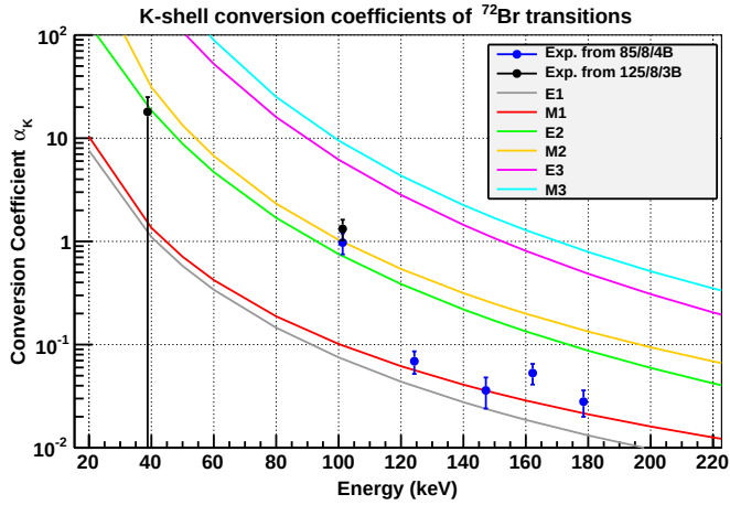
Figure E.8: Coeficientes de conversión experimentales para transiciones de electrones de capa K obtenidas con las configuraciones 85/8/4B y 125/8/3B del espectrómetro de electrones. La comparación se hace con las predicciones teóricas tomadas de Ref. [ANU] para las diferentes multipolaridades.
