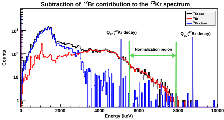
Figure E.3: Sustracción de la contribución de la desintegración de ^{72}\text{Br} al espectro de la medida del fichero 1 de la desintegración de ^{72}\text{Kr} . La región considerada para la normalización se muestra indicada y es elegida entre los valores Q_{CE} de la desintegraciones de ^{72}\text{Kr} y ^{72}\text{Br} . En esta región energética se espera encontrar únicamente contribución procedente de la desintegración de ^{72}\text{Br} .
