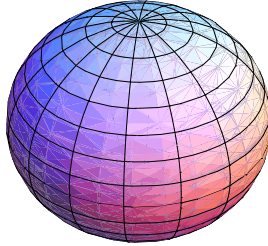
Figure E.12: Forma del núcleo ^{72}\text{Kr} en su estado fundamental obtenida con un parámetro de deformación cuadrupolar \beta_2=-0.1759 como sugiere P. Sarriguren en [Sar09a]. Este estado se corresponde con la deformación oblada cuya distribución de B(GT) teórica se representa en la figura E.11 en azul y que reproduce bastante bien la distribución hallada experimentalmente.
