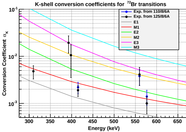
Figure E.10: Coeficientes de conversión experimentales para transiciones de electrones de capa K obtenidos con las configuraciones 110/8/6A y 125/8/6A del espectrómetro de electrones. La comparación se hace con las predicciones teóricas tomadas de Ref. [ANU] para las diferentes multipolaridades.
