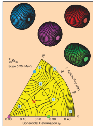
Figure E.2: Superficies de energía potencial para ^{72}\text{Kr} con respecto a los parámetros de deformación \varepsilon_2 y \gamma obtenidos de cálculos macroscópicos-microscópicos realizados en [Mð09]. Las líneas equipotenciales están distanciadas 0.2 MeV. Los números indican la energía en MeV de la línea sobre la que aparecen. Varios mínimos de energía se encuentran para este caso, indicados con marcadores azul, verde, rojo y violeta, que se corresponden con las formas del núcleo representadas en la parte superior de la figura en los mismos colores que los marcadores a que corresponden. Esta variedad de deformaciones para mínimos locales que se encuentran próximos en energía constituye lo que se denomina coexistencia de formas.
