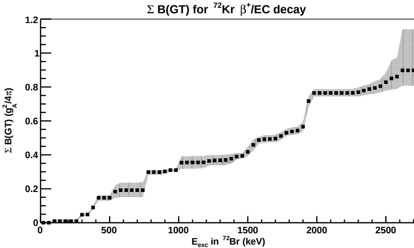
Figure E.6: Distribución de B(\text{GT}) acumulada para la desintegración \beta^+/\text{CE} de ^{72}\text{Kr} obtenida del presente análisis de la componente \beta^+ a través de Espectroscopía de Absorción Total (TAS). La región de incertidumbre mostrada está estimada a partir de origen estadístico y sistemático como se describe en el texto.
