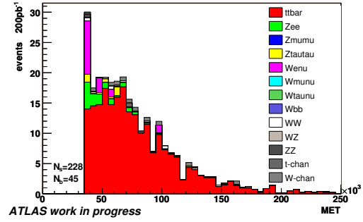
(d) Selected E_{t,miss} distribution.
