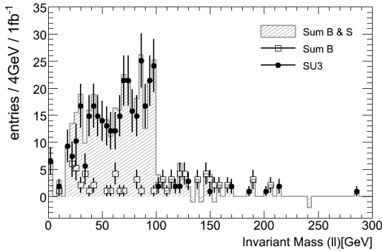
(d) M_{\text{eff}} > 800 \text{ GeV}
