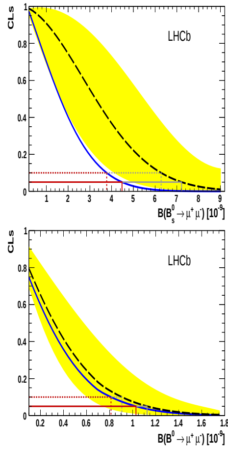
Figure 0.10: CL_s en fonction de B(B_s^0 \rightarrow \mu^+ \mu^-) . La ligne noire en pointillés correspond à la médiane des valeurs du CL_s , tandis que la zone jaune couvre la région de 68% compatibilité avec la valeur moyenne. La ligne bleue correspond à la CL_s observée. Le 90% CL et 95 % sont donnés par l'horizontale en pointillés et solides lignes rouge, respectivement.
