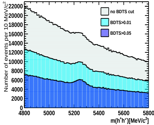
Figure 0.5: Distribution de la masse invariant des événements B_{(s)}^0 \rightarrow h^+h'^- TIS pour différents selections en BDTS.
