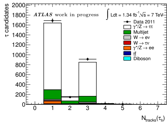
(d) \tau_e\tau_h channel.
