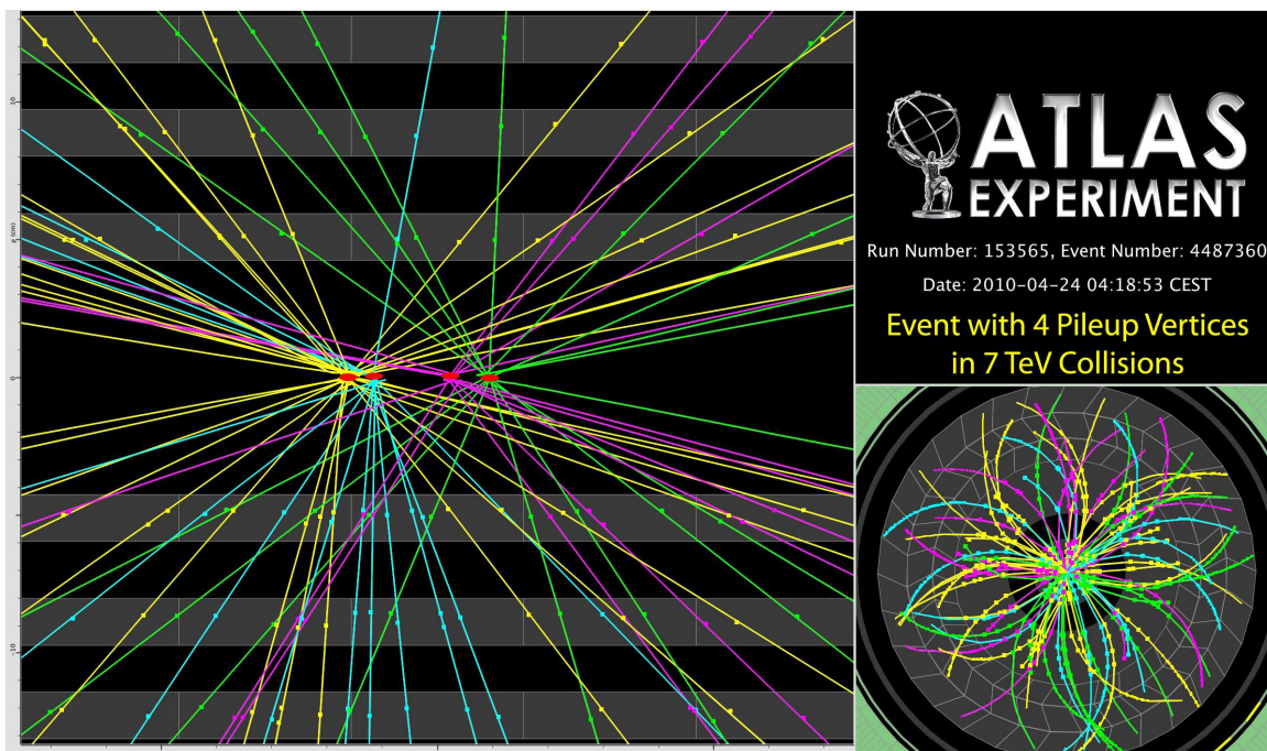
FIG. 6.14 – Empilement de quatre collisions reconstruites par ATLAS, et séparées grâce au détecteur à pixels.
