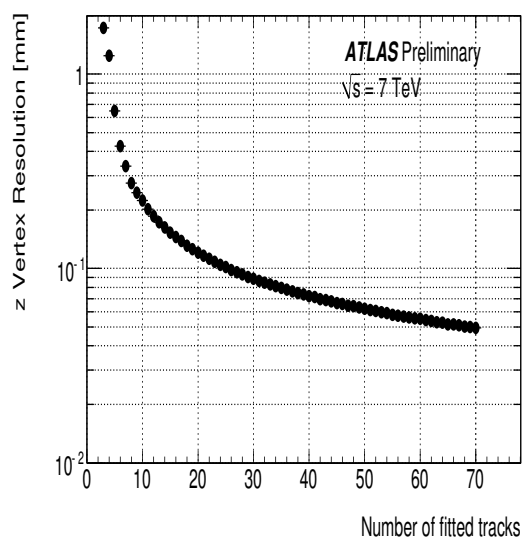
FIG. 6.16 – Résolution sur la position longitudinale du vertex primaire en fonction du nombre de particules chargées qui en sont issues.
