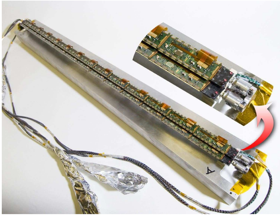
FIG. 6.4 – Double échelle du détecteur à pixels d’ATLAS. On distingue les treize modules qui forment chacune des échelles.
