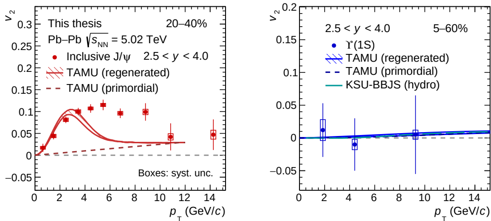
Figure D.1: Comparaison des v_2 du J/\psi (left) et de l' \Upsilon(1S) (right) dans les collisions Pb–Pb non-centrales, avec différents modèles théoriques qui incluent différentes fractions de régénération et/ou suppression.
