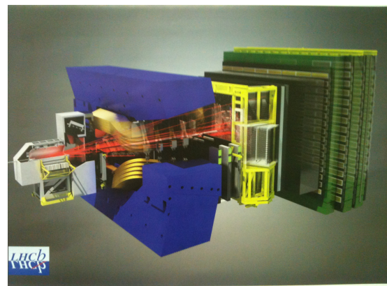
(b) LHCb.
