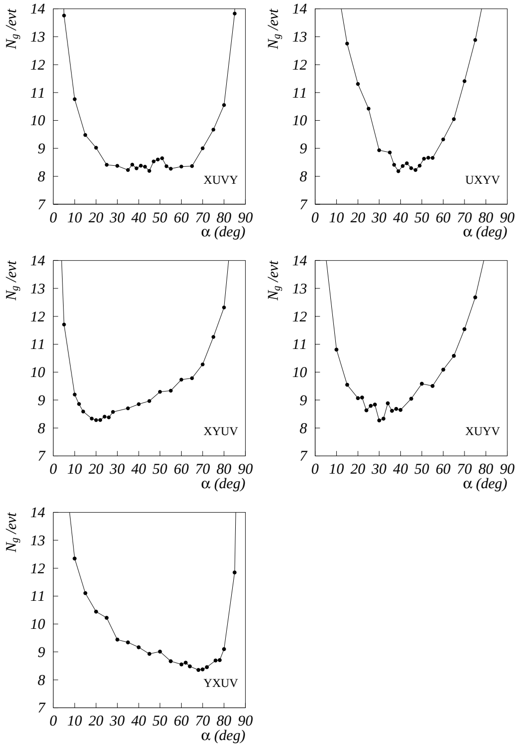
Figure 5.12: Nombre moyen de traces fantômes par événement pour différentes configurations d'une station de chambres à dérives, en fonction de l'orientation \alpha des chambres inclinées.
