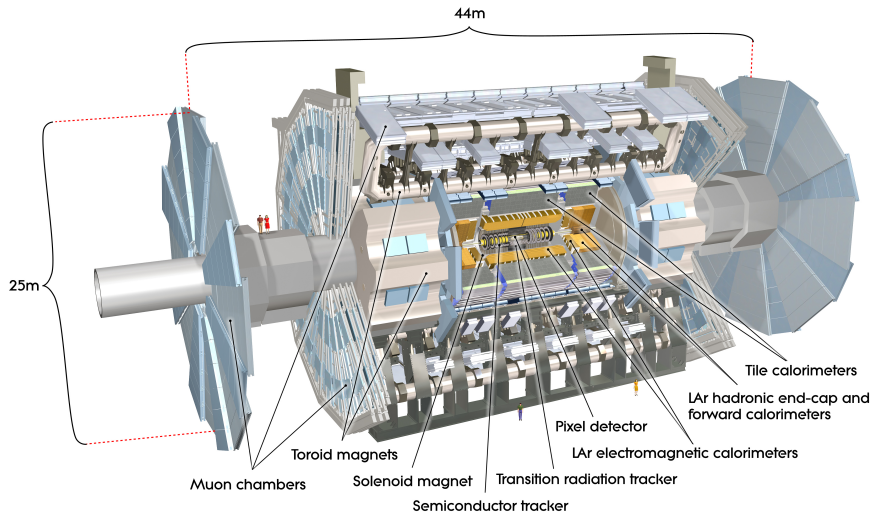
Figura 18.2: Vista axial del detector ATLAS, mostrant els seus principals components: les cambres de muons, els calorímetres electromagnètic i hadrònic, el Detector Intern i els sistemes d'imants: toroide i solenoide [29].
