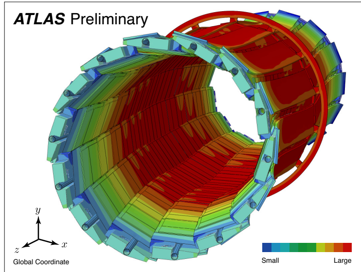
Figura 18.7: Simulació mitjançant un anàlisi d'elements finits del IBL. Els resultats de la simulació coincideixen amb l'arquejament de les dogues del IBL tal com s'ha observat a l'alinejar el detector real. [61]
