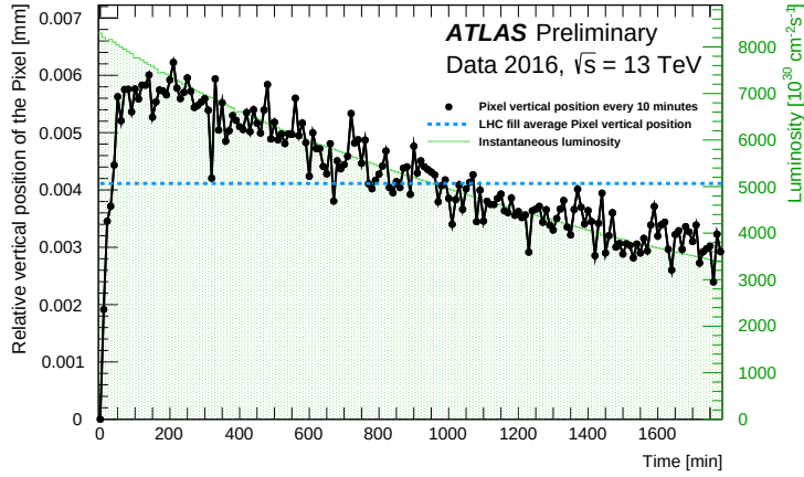
Figura 18.5: Moviments verticals del detector Pixel durant un run d'ATLAS. Existeixen dos components diferents: durant la primera hora prenent dades, el Pixel s'eleva ràpidament varies micres. Després d'este primer desplaçament, el Pixel descendeix lentament durant la resta del run. La velocitat de la segona component mostra una alta correlació amb la lluminositat instantània del run [59].
