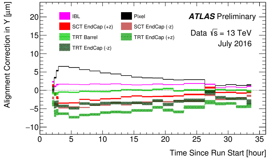
Figura 18.9: Correccions a la posició vertical en funció del temps, de les estructures que componen l'ID. Mencionar que el barril del SCT defineix la referència i per tant es manté fixa. Les bandes que acompanyen les línies mostren la incertesa estadística [58].
