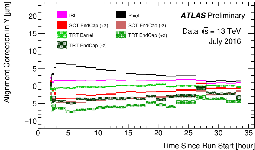
Figura 17.9: Correcciones a la posición vertical de los componentes del ID en función del tiempo. El barril del SCT se mantiene fijo como referencia. Las bandas indican la incertidumbre estadística [58].
