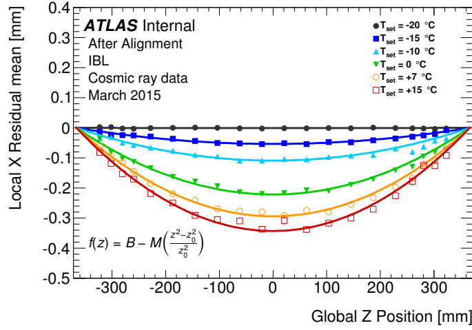
Figura 17.6: La media de los residuos traza-síñal en función de la posición de los detectores a lo largo de la duela del IBL. Para cada posición, se hace la media de las catorce duelas que componen el IBL. Se ha realizado un ajuste a cada distribución utilizando una función parabólica [61].
