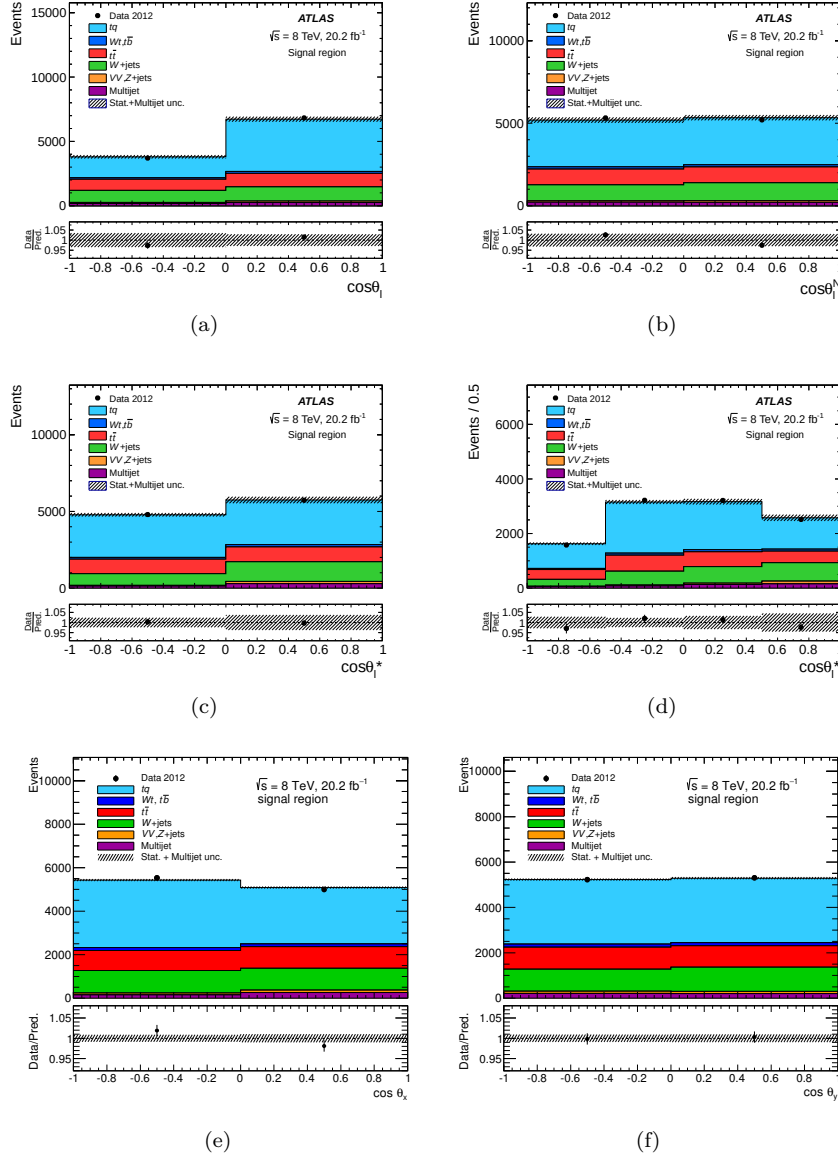
Figura 17.13: Distribuciones angulares en la región de señal (a) \cos \theta_\ell , (b) \cos \theta_\ell^N , (c) \cos \theta_\ell^* con 2 bins y (d) \cos \theta_\ell^* con 4 bins, (e) \cos \theta_x y (f) \cos \theta_y . Electrones y muones han sido combinados.
