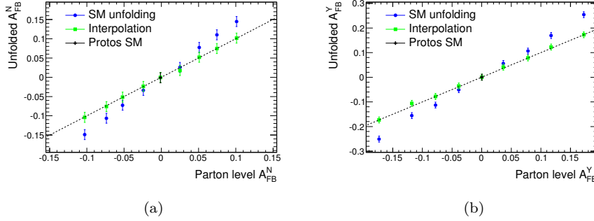
Figura 18.14: Valor deconvolucionat d'(a) A_{FB}^N i (b) A_{FB}^Y en funció del valor generat per l'asimetria. La deconvolució s'ha fet o bé directament amb les correccions del SM (punts blaus) o amb el mètode d'interpolació (quadrats verds). Les barres d'error representen la incertesa deguda a la limitada estadística de les mostres. La línia puntejada està per indicar el cas de linealitat perfecta.
