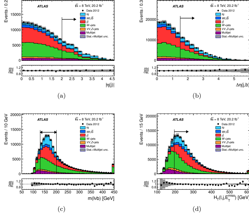
Figura 18.10: Distribucions dels observables emprats en la selecció del senyal partint dels esdeveniments preseleccionats (el veto al segon leptó ja està sent aplicat). Les línies verticals delimiten el tall per seleccionar el senyal. (a) pseudorapidesa del quark espectador, (b) diferència en pseudorapidesa d'ambdós jets, (c) massa reconstruïda del quark top, i (d) suma de la massa transversa de tots els objectes reconstruïts.
