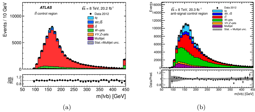
Figura 17.11: Distribución de la masa reconstruida del quark top en las regiones de control t\bar{t} (a) y anti-señal (b) para electrones y muones combinados.
