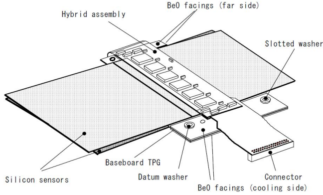
Figure 2.10: SCT module structure [28].
