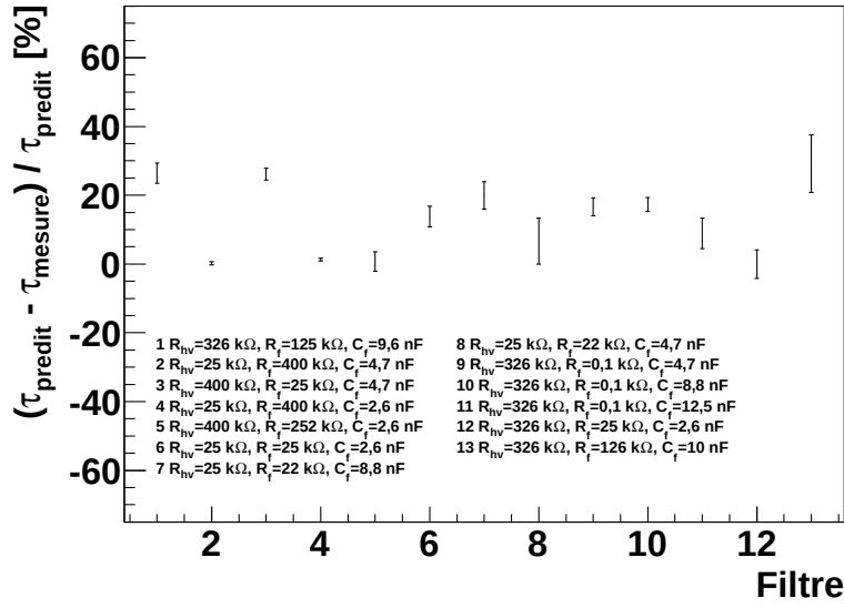
FIGURE 3.6 – Comparaison des constantes longues prédite et mesurée en fonction du filtre. La capacité du détecteur est ajustée à C_{mg} = 1,2 nF. Une grande barre d'erreur indique que la constante de temps varie beaucoup d'une mesure à l'autre.
