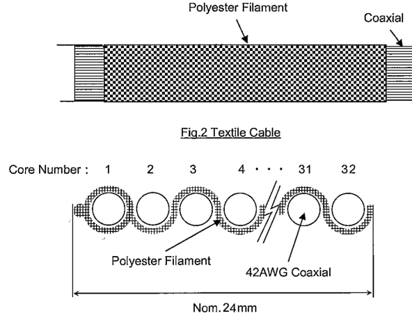
FIGURE 4.3 – Schéma d'une limande coaxiale tissée.
