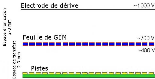
FIGURE 1.12 – Schéma de principe d'un détecteur GEM.
