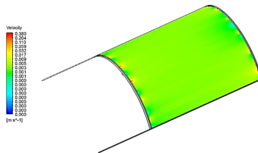
FIGURE 6.14 – Simulation par éléments finis avec le logiciel OpenFoam de la vitesse de déplacement du gaz dans un détecteur courbe, lorsque ce dernier est équipé d'une zone tampon [69].
