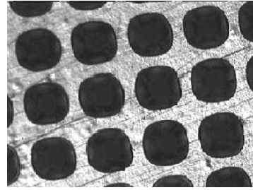
FIGURE 1.13 – Vue au microscope d'une feuille de GEM.
