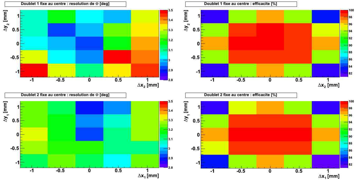
FIGURE 7.13 – Résolution en \phi et efficacité en fonction du désalignement. Les figures du haut concernent la résolution en \phi et l'efficacité en fonction du déplacement du deuxième doublet, le premier doublet étant fixe et aligné avec le champ magnétique. Les figures du bas présentent les mêmes paramètres en inversant les rôles des doublets.
