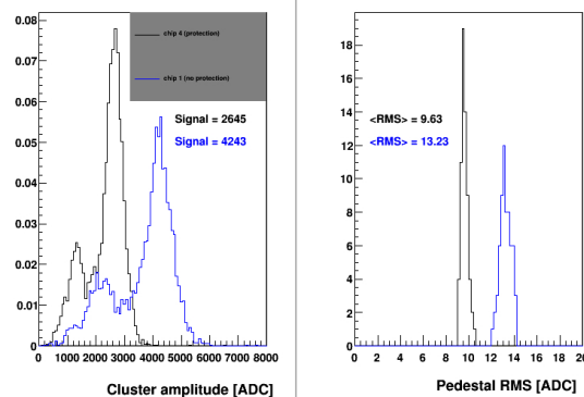
FIGURE 6.11 – Amplitude du signal (à gauche) et bruit (à droite) du RTF10 lorsqu’une source de ^{55}\text{Fe} est posée sur le détecteur selon que l’électronique est équipée d’un circuit de protection (courbe noire) ou non (courbe bleue).
