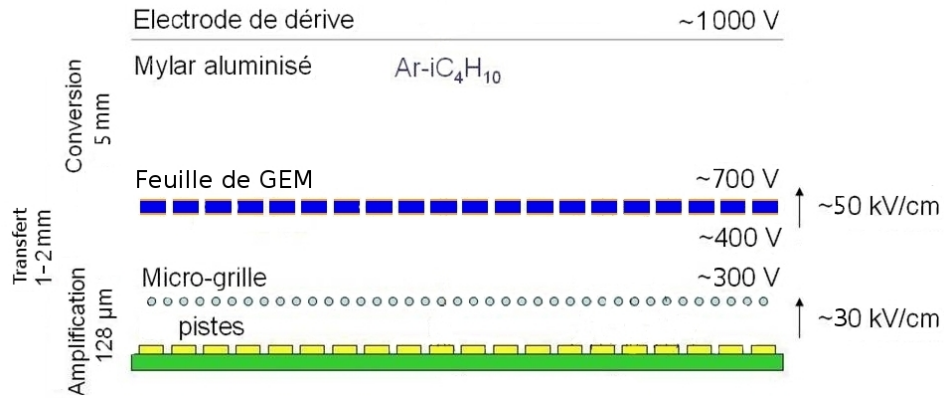
FIGURE 3.15 – Vue en coupe d'un Micromegas avec une feuille de GEM placée entre la dérive et la microgrille.
