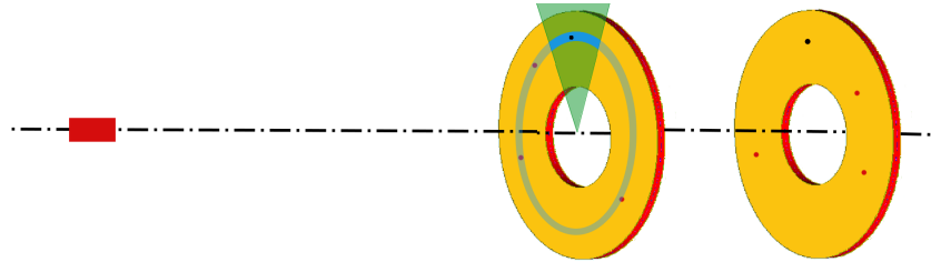
FIGURE 7.9 – Illustration des coupures du FT-Trck. Le cône vert représente la coupure en \phi et la section de disque en bleu pâle la coupure en \theta . Sur la première couche une surface de correspondance (en bleu) est alors définie par la position du cluster (point noir) de la seconde couche.
