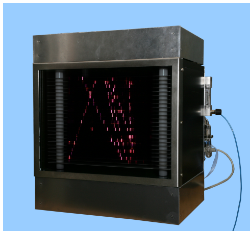
FIGURE 1.5 – Photographie d'une chambre à étincelles en fonctionnement (Université de Cambridge).
