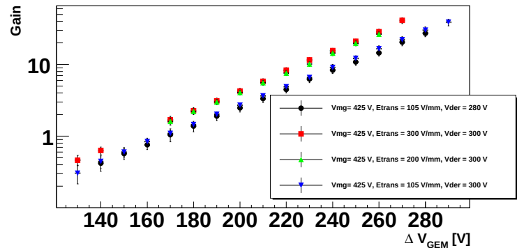
FIGURE 3.19 – Gain de la feuille de GEM en fonction de la différence de tension entre ses deux faces pour différents champs.
