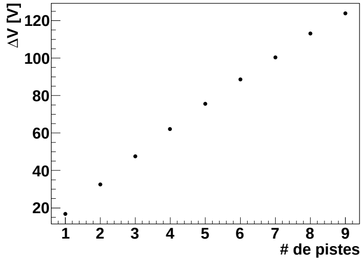
FIGURE 3.11 – \Delta V en fonction du nombre de pistes impliquées dans la décharge lorsque la capacité d'une piste est de 74 pF. Les simulations sont réalisées avec LTSpice.
