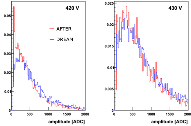
FIGURE 4.5 – Distributions de l’amplitude du signal créé par des particules cosmiques pour le CR6-Z à différentes tensions lorsque le détecteur est connecté à l’électronique Dream ou After. On remarque la différence de bruit entre les deux électroniques sur le graphe de gauche. Le mélange gazeux est de l’argon-isobutane à 5 %.
