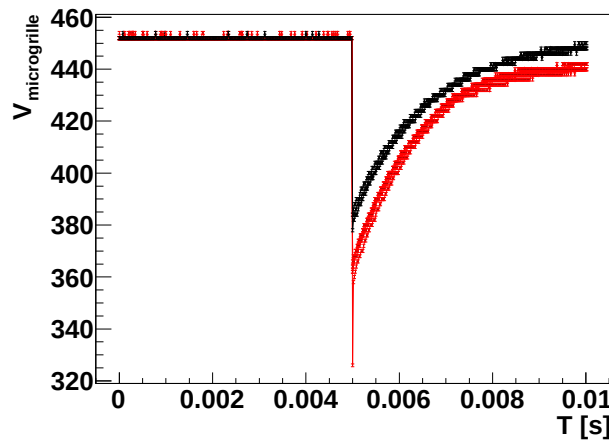
FIGURE 3.5 – Remontées en tension après une décharge dans le TF10. Les courbes dont la constante de temps diffère de plus de 20 % de la constante prédite sont en rouge.
