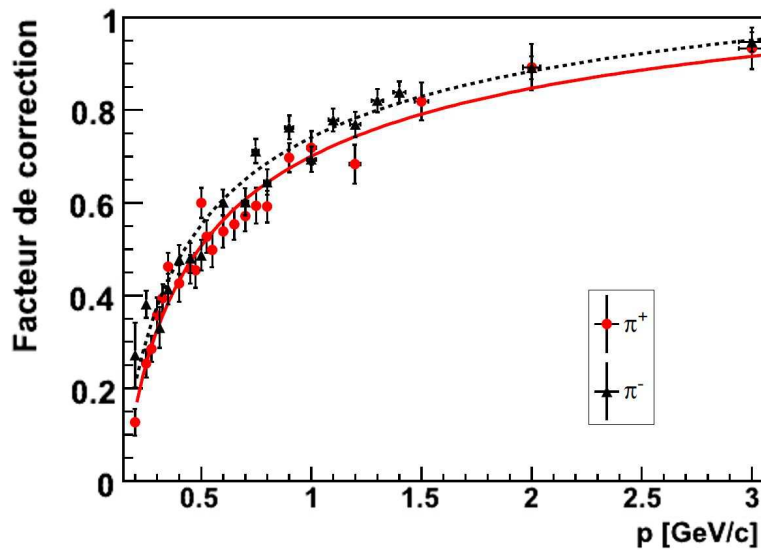
FIGURE 3.25 – Facteur de correction de la luminosité en fonction de l'impulsion d'un détecteur pour des \pi^+ et des \pi^- . Les courbes continues sont des ajustements qui sont ensuite utilisés pour les calculs de probabilité de décharges.
