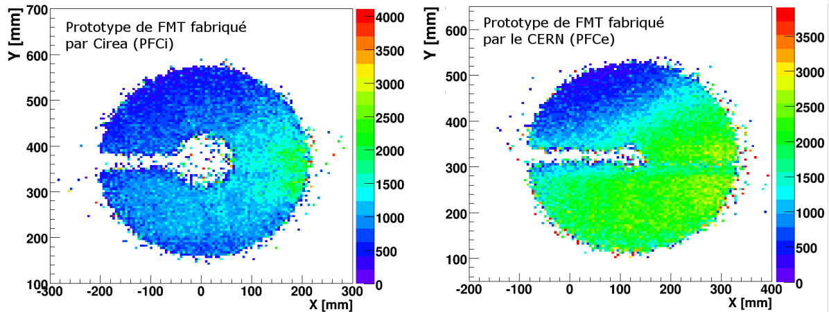
FIGURE 6.16 – Amplitude maximale du signal des deux prototypes de FMT dans un mélange d’argon-isobutane à 5 % dont le débit est d’environ 2 L/h. La tension de la microgrille est de 450 V et celle de la dérive de 750 V.
