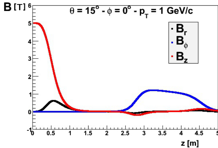
FIGURE 2.20 – Champs magnétiques radial, azimuthal et longitudinal en fonction de la coordonnée selon l'axe du faisceau subis par un proton de 1 GeV/c émis de la cible à 15^\circ .
