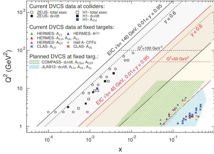
FIGURE 2.11 – Domaines cinématiques des expériences existantes et prévus pour la mesure de réactions DVCS [48].
