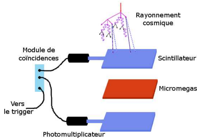
FIGURE 1.19 – Schéma de principe d'un banc cosmique.
