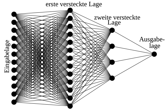
Abbildung 5.6: Netzwerktopologie bei der (h)q\bar{q} -Suche
