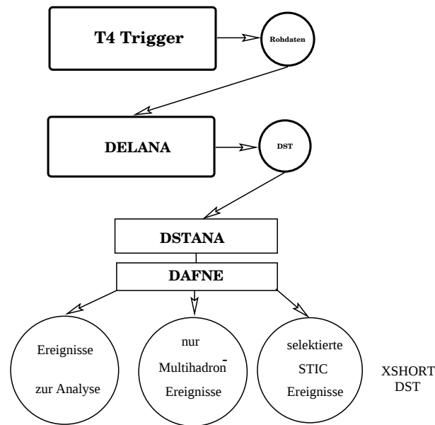
Abbildung 3.9: Der Offline-Datenstrom
