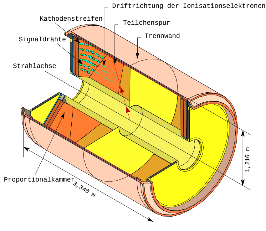
Abbildung 3.7: Die Hauptspurkammer TPC
