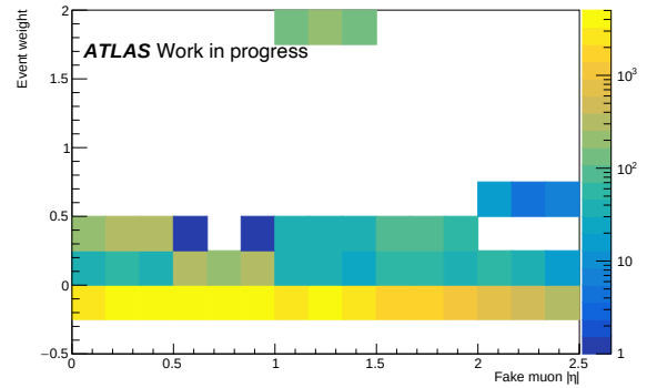
(b) Muons
