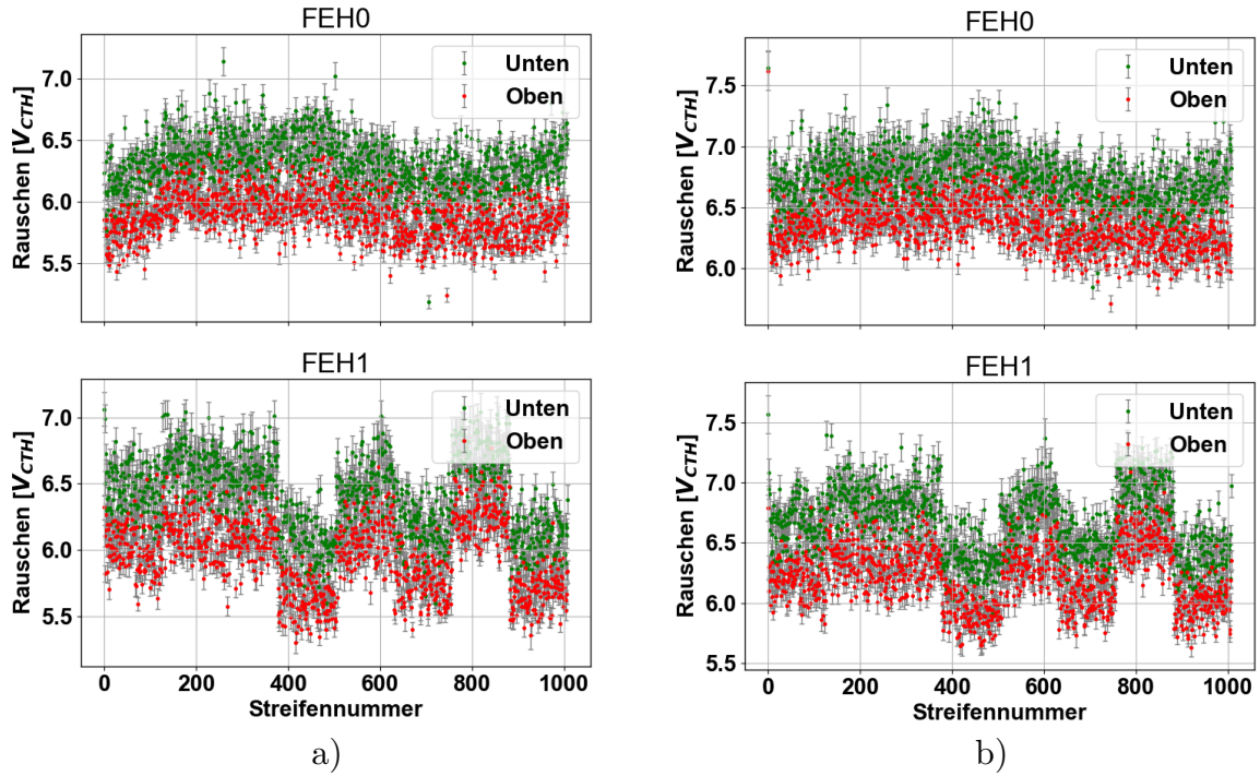
Abbildung 24: Rauschen im Modul mit Regular Design SEH a) mit angeschlossenem Ground Balancer und b) ohne.
