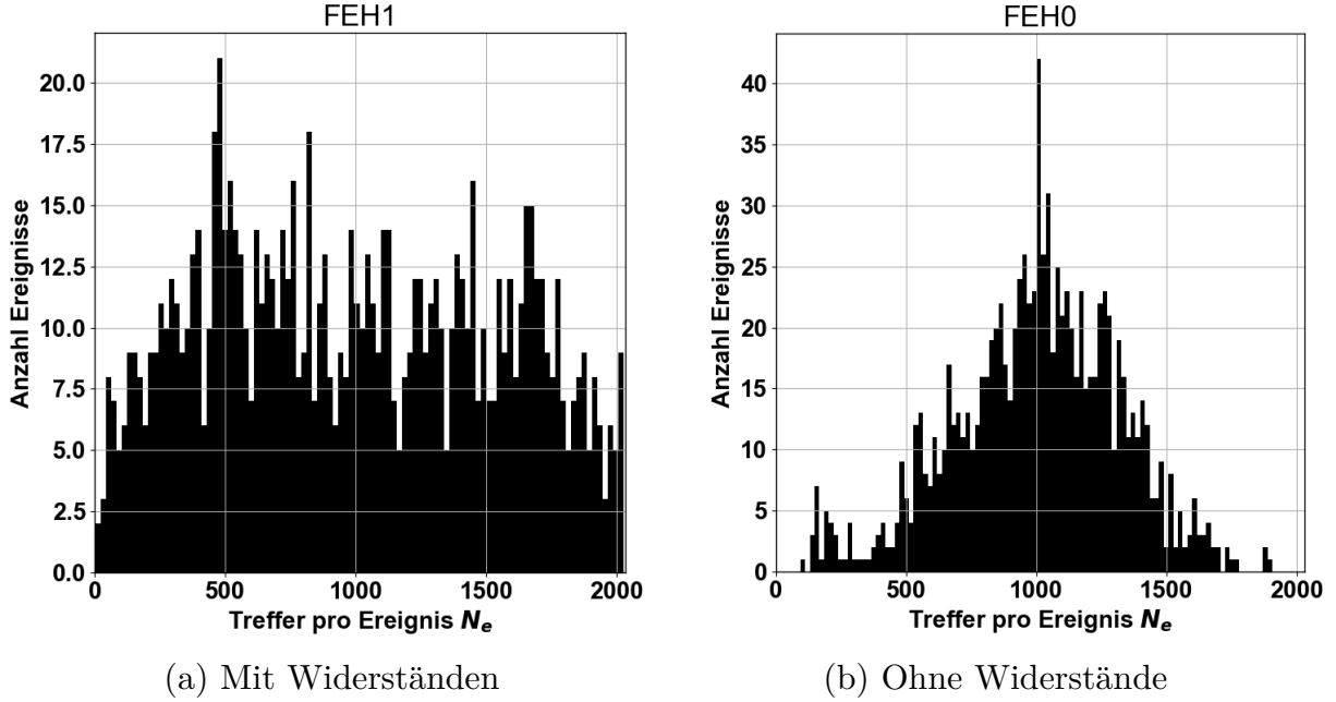
Abbildung 37: Histogramme der Trefferanzahl pro Ereignis für die Messungen mit dem Prototypmodul mit Widerständen in den HV-Tails und ohne.
