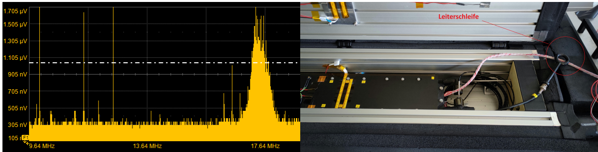
Abbildung 49: Frequenzspektrum der im Labor gemessenen 17.5 MHz Strahlung (links) und Messung der Strahlung mit einer Leiterschleife an den Kabeln der, in der Mini-TEDD verbauten Temperatursensoren (rechts).
