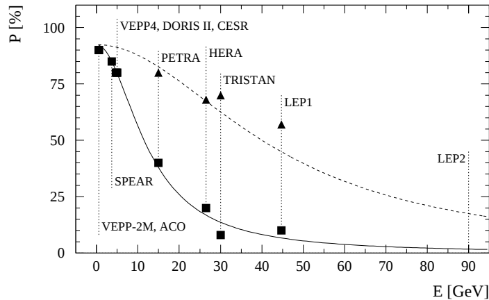
Abbildung 5.15: Die maximal gemessene transversale Polarisation P wird für verschiedene Speicherringe ohne (Quadrate) und mit (Dreiecke) harmonischer Spin-Orbitkorrektur verglichen. Die Messungen von SPEAR und HERA wurden unter Benutzung von Gl. 5.13 mit der Strahlenergie E extrapoliert (Kurven). Dabei wurde angenommen, daß die Speicherringe die gleichen Unvollkommenheiten aufweisen und daß die lineare Approximation gültig ist.
