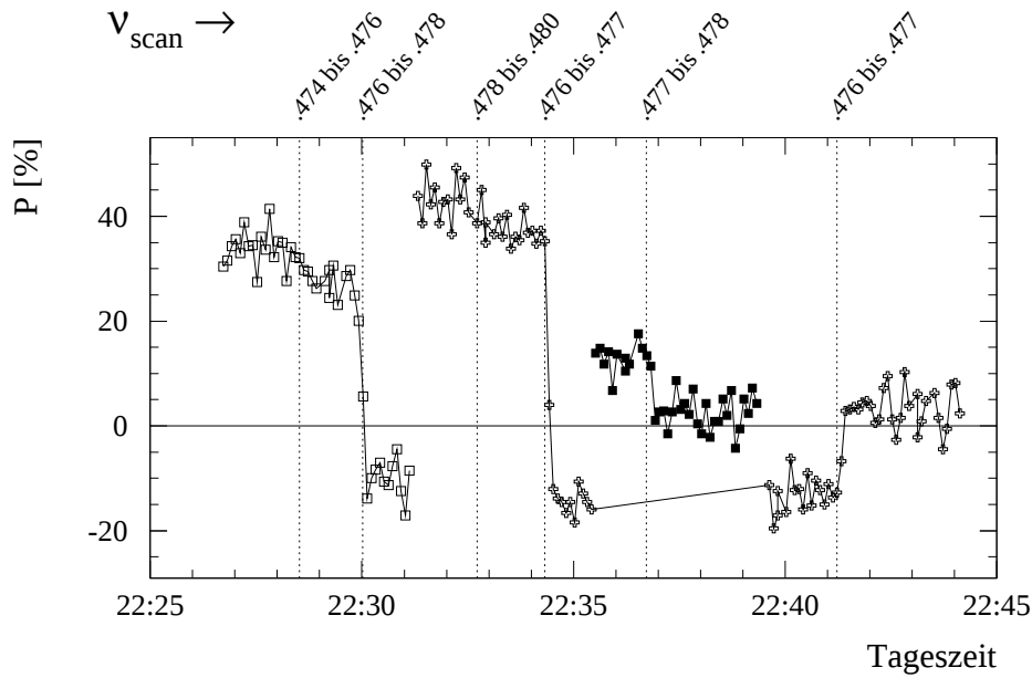
Abbildung 6.1: Messung der Spinzahl \nu . Die Spinpräzession wurde auf drei verschiedenen Teilchenpaketen durch ein mit der Frequenz \nu_{\text{scan}} oszillierendes Dipolfeld gestört. Für \nu_{\text{scan}} \approx [\nu] wurden resonante Spinvektordrehungen beobachtet. Dabei wurde ein teilweises Umklappen des Polarisationsvektors beobachtet. In der letzten Messung konnte der zuvor umgeklappte Polarisationsvektor erneut teilweise umgeklappt werden.
