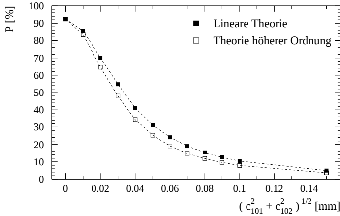
Abbildung 3.9: Berechnete Abhängigkeit des Polarisationsgrades P von der Stärke c_k der beiden nächsten Ganzzahl-Spinresonanzen. Die Rechnung wurde für eine Spinzahl von 101.47 mit SODOM durchgeführt.
