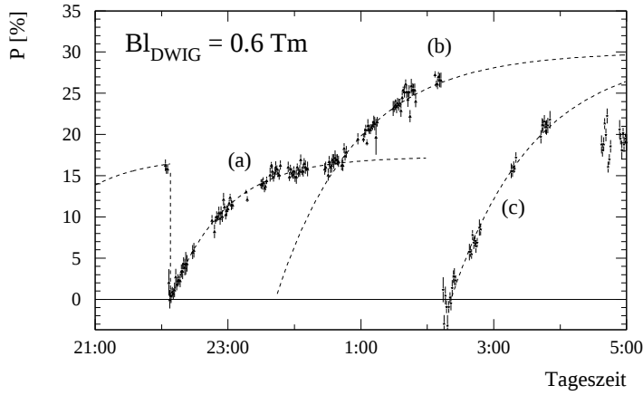
Abbildung 5.23: Polarisationsaufbau mit den Dämpfungswiggeln auf je 0.6 Tm. Die drei verschiedenen Kurven wurden mit verschiedenen Teilchenpaketen gemessen. Nach einer zweiten Stufe deterministischer harmonischer Spin-Orbitkorrektur wurde eine Polarisation von 30% erreicht.
