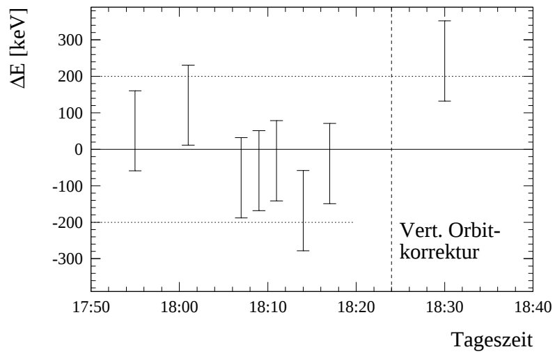
Abbildung 6.5: Stabilität der auf den acht verschiedenen Elektronenpaketen gemessenen Strahlenergie. Für jede Messung ist der Bereich \Delta \nu_{\text{scan}} angegeben, in dem die Energie gefunden wurde (Balken). Die gepunktete Linien geben den erwarteten systematischen Fehler wieder.
