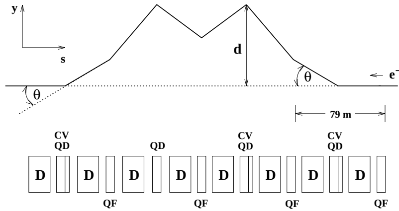
Abbildung 3.3: Schematische Darstellung einer geschlossenen Beule im vertikalen Gleichgewichtsort. Der Phasenvorschub in der vertikalen Ebene beträgt 60^\circ pro Standardzelle von 79 m. Insgesamt erstreckt sich die Orbitbeule über \pi ( = 237 m). An zwei vertikalen Korrekturspulen (CV) wird der Teilchenstrahl ausgelenkt. An den fokussierenden und defokussierenden Quadrupolen (QF und QD) erfährt er innerhalb der Beule zusätzliche Ablenkungen. Dipolmagnete (D) mit vertikalem Feld halten die Teilchen auf einer Kreisbahn und führen zur Spinpräzession um die vertikale Richtung. In der Darstellung sind Sextupole, Strahlpositionsmonitore und vertikale Korrekturspulen ausgelassen.
