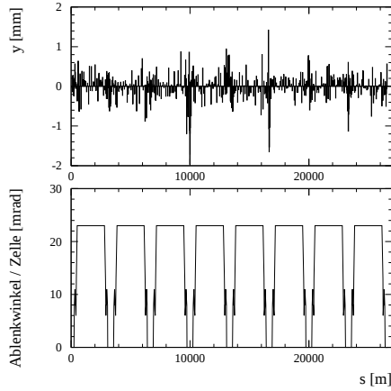
Abbildung 5.7: Oben: Gemessener vertikaler Gleichgewichtsortbit. Unten: Der Ablenkwinkel ist die periodische Variable der Fourieranalyse.
