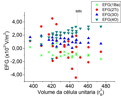
Fig. 4.13 b) V_{zz} medido nas posições 1Ba, 2Ti, 3O e 4O, em função do volume para o sistema com os átomos nas posições relativas da fase ferroelétrica após ter sido efectuada a relaxação do sistema.
