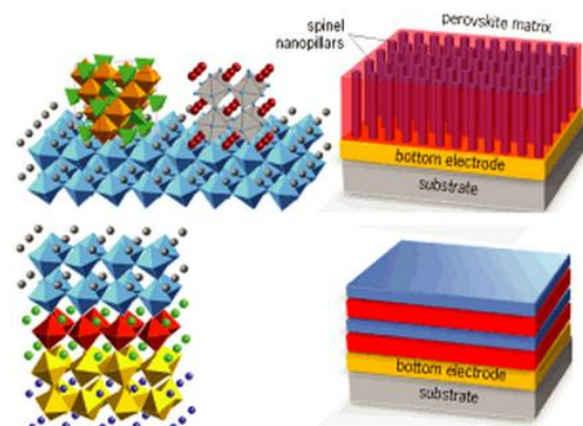
Fig. 2.4 - Modelo atômico (esquerda) e macroscópico (direita) de heteroestruturas multiferróicas [10].
