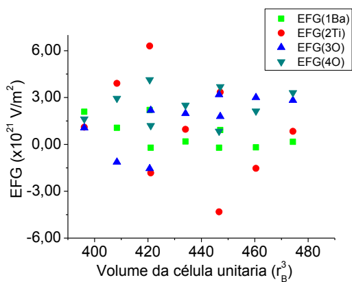
Fig. 4.13 a) V_{zz} medido nas posições 1Ba, 2Ti, 3O e 4O, em função do volume, para o sistema com os átomos nas posições relativas da fase paraelétrica.
