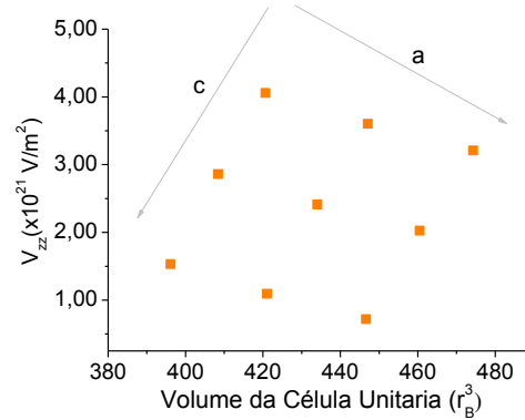
Fig. 4.11 b) Representação da rede de pontos do V_{zz} medido na posição do oxigênio, (30), em função do volume, com os átomos nas posições relativas da fase ferroelétrica.
