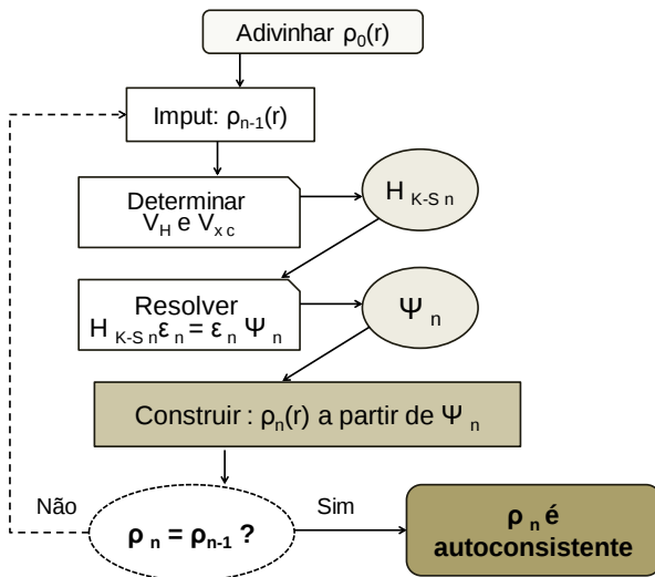
Fig. 4.1 a) Fluxograma do método autoconsistente, relativo à iteração n , para resolver as equações de Kohn-Sham.
