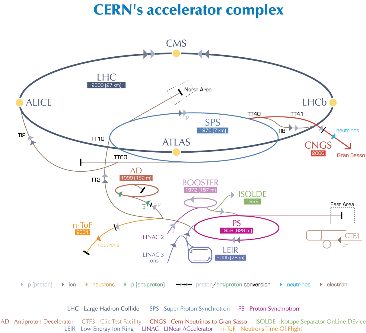
FIGURE 2.2 – Schéma de l’organisation du complexe d’accélérateurs du CERN. ©CERN
