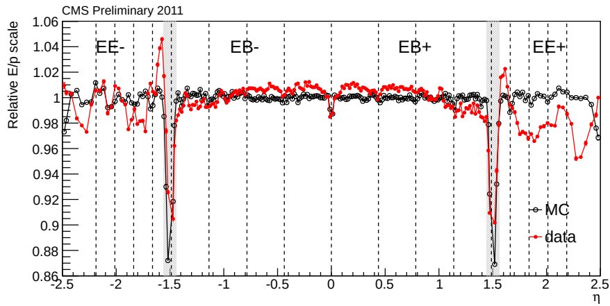
FIGURE 3.19 – Échelle relative E/p issue des désintégrations W \rightarrow e\nu en fonction de la pseudo-rapacité \eta . Figure tirée de [68]
