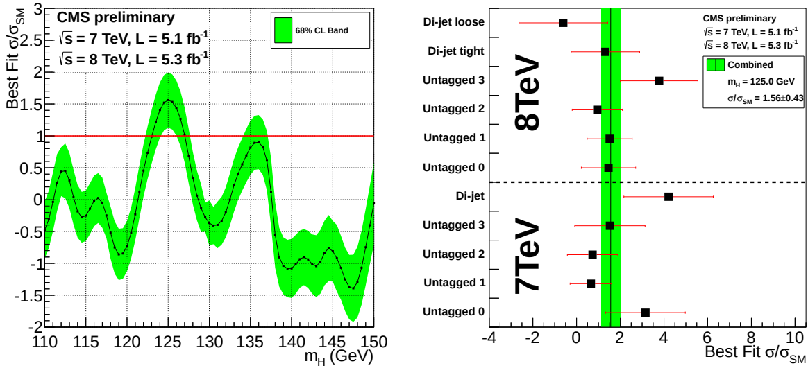
(a) Meilleur ajustement de la force du signal en fonction de m_H . (b) Meilleur ajustement de la force du signal à l'hypothèse de masse m_H = 125 \text{ GeV} pour chaque classe d'événements.
