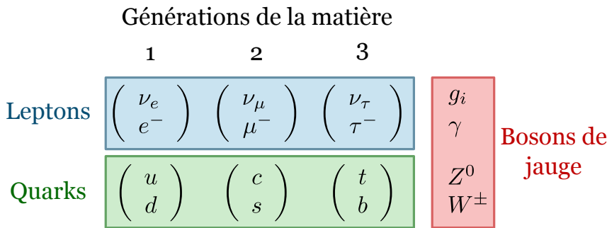
FIGURE 1.1 – Les particules du Modèle Standard. Les fermions (de spin 1/2) sont regroupés en trois générations (ou familles), et en deux ensembles : les leptons, soumis aux interactions faible et électromagnétique, et les quarks, soumis aux interactions faible, électromagnétique et forte. Les bosons de jauge (de spin 1) sont les particules agissant comme porteurs des interactions. Les gluons g_i portent l’interaction forte, le photon \gamma porte l’interaction électromagnétique et les bosons W^\pm et Z^0 portent l’interaction faible.
