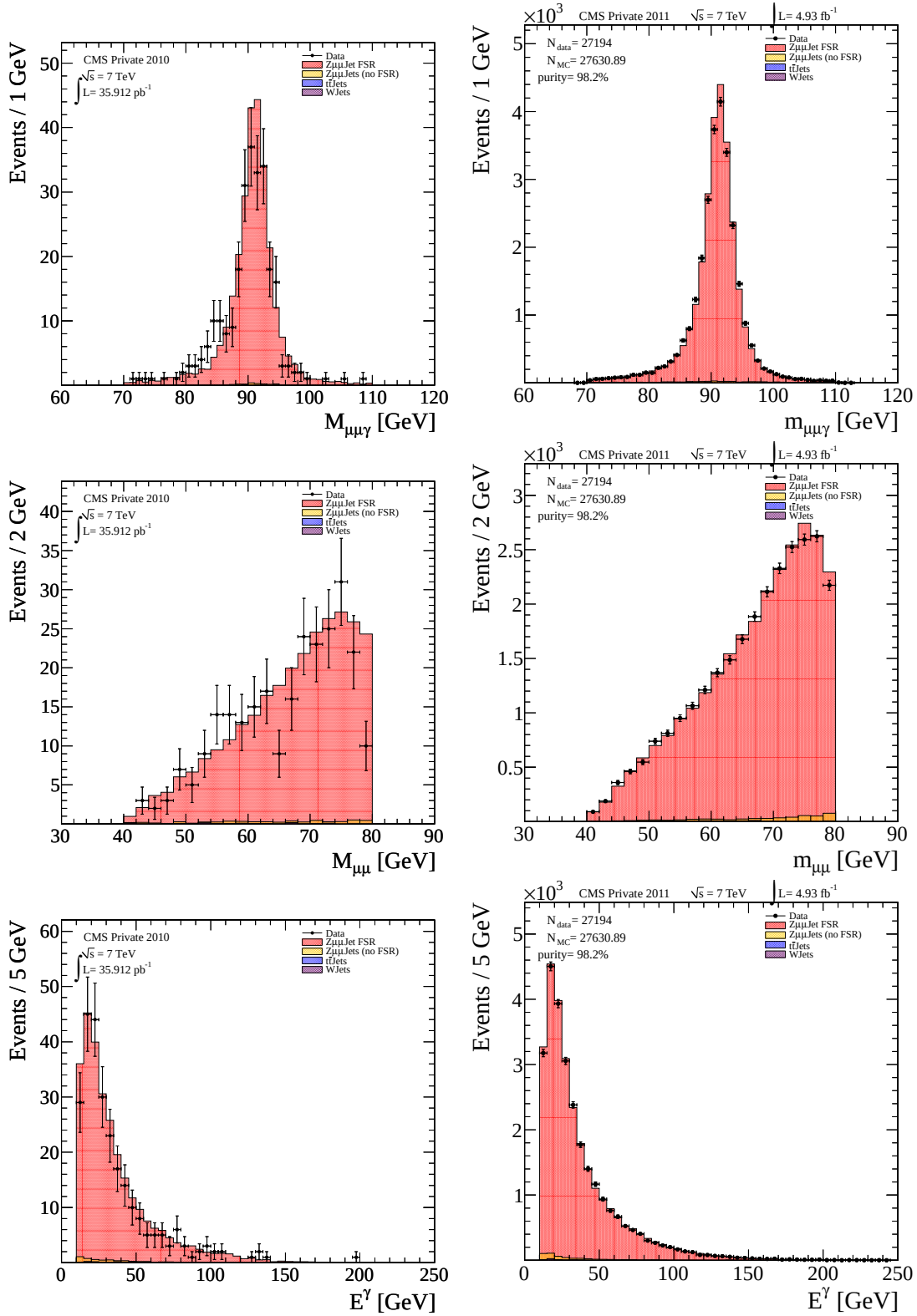
FIGURE 4.4 – Comparaisons données simulation pour les données 2010 (gauche) et les données 2011 avec la calibration du 16 janvier (droite), illustrant quelques variables cinématiques des désintégrations radiatives : masse invariante à trois corps m_{\mu\mu\gamma} (haut), masse invariante du système dimuon m_{\mu\mu} (milieu) et énergie du photon E^\gamma (bas).
