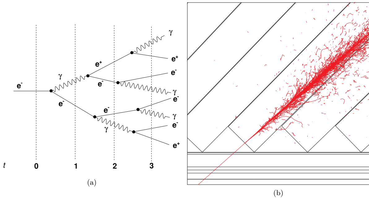
FIGURE 3.2 – Principe de développement d'une gerbe électromagnétique (gauche, tirée de [60]) et simulation d'une gerbe dans les cristaux de CMS (droite, tirée de [43]).
