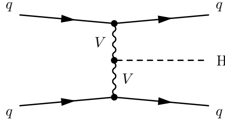
FIGURE 1.9 – Production d'un boson de Higgs par fusion de boson vecteurs (VBF), en association avec deux quarks.
