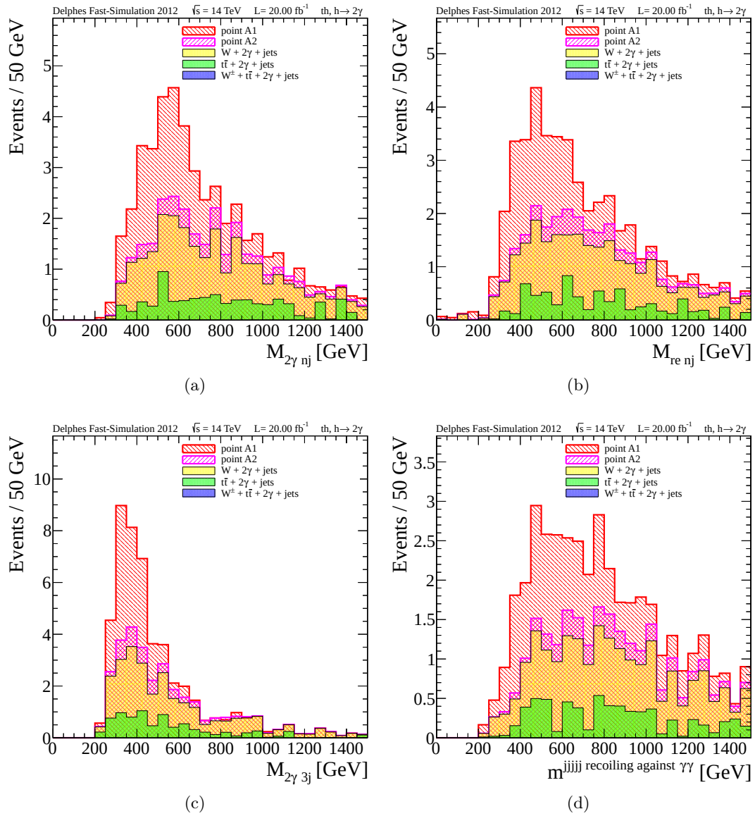
FIGURE 6.8 – Distributions de la masse invariante des deux hémisphères, côté Higgs M_{2\gamma nj} (a) et côté recul M_{re nj} (b) après l'ensemble des critères de sélection, calculées selon l'algorithme présenté à la section 6.4.2. Les figures (c) et (d) montrent respectivement la masse invariante du système diphoton et des trois jets les plus proches, et la masse invariante des cinq jets les plus éloignés du système diphoton. On peut rappeler (voir table 6.2) que m_{t_2} = 403 GeV dans le cas du point A1 et m_{t_2} = 599 GeV dans le cas du point A2. La somme des distributions du signal et du bruit de fond est normalisées à 20 fb ^{-1} .
