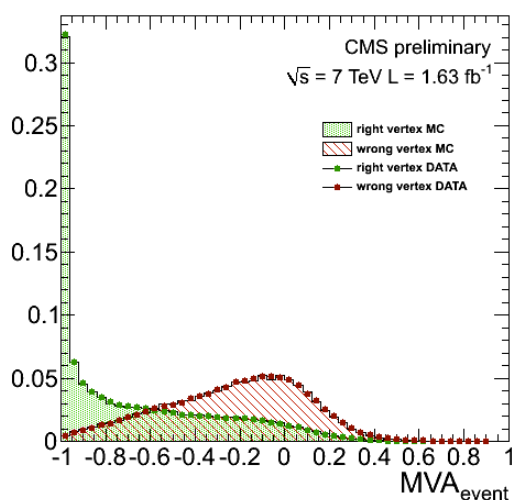
FIGURE 5.4 – Sortie de l’arbre de décision boosté de probabilité d’avoir choisi le mauvais vertex pour des événements de désintégration Z^0 \rightarrow \mu^+ \mu^- , dans lesquels les muons ont été enlevés. Une valeur de sortie de l’arbre de -1 correspond donc à une haute probabilité d’avoir choisi le bon vertex. On observe un bon accord entre données et simulation. Figure tirée de [91].
