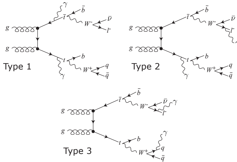
FIGURE 6.2 – Diagrammes de Feynman illustrant les trois types de radiations dans l'état final dans les événements t\bar{t} + jets dans l'analyse t\bar{t}H, H \rightarrow \gamma\gamma du Technical Design Report de l'expérience CMS [104]. Les photons à l'état final peuvent soit provenir des radiations des quarks top dans l'état final (Type 1), soit des radiations des produits de désintégrations des quarks top (Type 3), soit d'une combinaison de ces deux types (Type 2). Par défaut dans Alpgen, seul le type 1 est inclus, tandis que pour l'analyse de ce Technical Design Report, une version privée, développée par les auteurs d'Alpgen, a été utilisée. Le développement d'Alpgen a continué par la suite, et cette version privée n'est plus compatible avec la dernière version d'Alpgen (notamment à cause de changements dans la syntaxe des cartes de génération). Il n'a pas été possible techniquement d'inclure cette ancienne version privée d'Alpgen dans la dernière version. On sait cependant grâce à cette analyse t\bar{t}H, H \rightarrow \gamma\gamma que l'on peut sous-estimer la section efficace totale du processus \gamma\gamma + t\bar{t} + N jets de près de 90 %, lorsque les diagrammes de type 2 et 3 ne sont pas considérés. L'étude de l'interférence entre ces différents diagrammes, et l'étude d'un possible double comptage des photons avec ceux générés par le programme d'hadronisation (ici Pythia), devraient également être réalisées pour une modélisation correcte de ce processus.
