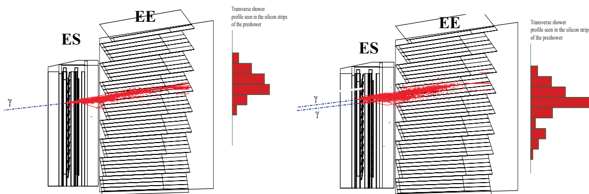
FIGURE 3.8 – Développement de gerbe électromagnétique dans le système bouchons et détecteur à pied de gerbe, dans le cas d'un photon (gauche) et de deux photons fortement collimatés provenant d'un pion neutre (droite). Le déclenchement prématuré de la gerbe par le détecteur à pied de gerbe étale le dépôt d'énergie et permet d'aider à distinguer les deux gerbes. Figure tirée de [60].
