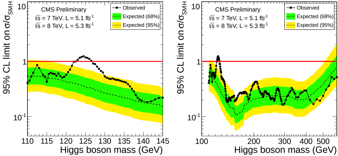
FIGURE C.1 – Limites d'exclusion pour la combinaison de l'ensemble des canaux de recherche du boson de Higgs du Modèle Standard dans l'expérience CMS, à basse masse (gauche) et pour l'ensemble des hypothèses de masse (droite). Figures tirées de [100].
