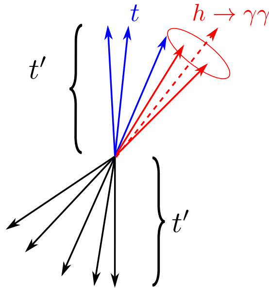
FIGURE 6.7 – Séparation des événements de signal en deux hémisphères.
