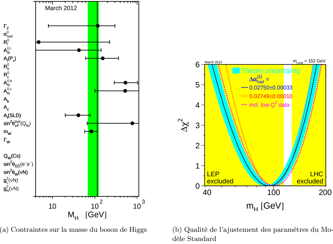
FIGURE 1.22 – Résultats de la combinaison des mesures de précision électrofaible du Tevatron, du LEP et du SLC. À gauche sont représentées les contraintes sur la masse du boson de Higgs pour différentes pseudo-observables. Ne sont représentées que les observables dont la précision de la mesure permet de contraindre la masse sur l'échelle de la figure. La bande verte représente la contrainte résultante à partir de toutes les pseudo-observables, la ligne verticale représente la limite expérimentale inférieure sur la masse du boson de Higgs à partir des recherches directes effectuées au LEP ( m_H > 114.4 GeV). À droite est représenté \Delta\chi^2 = \chi^2 - \chi_{\text{min}}^2 en fonction de la masse du boson de Higgs. La bande bleue représente l'incertitude théorique due aux corrections aux ordres supérieurs non inclus. Les bandes verticales représentent les limites d'exclusion directe des recherches effectuées au Tevatron et au LEP-II. La valeur préférée, correspondant au minimum de la courbe, correspond à m_H = 94^{+29}_{-24} GeV. Les figures sont de [33], mises à jour pour les conférences d'hiver 2012.
