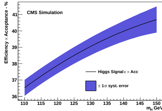
FIGURE 5.14 – Produit acceptance fois efficacité pour l’analyse présentée dans ce chapitre, en fonction de l’hypothèse de masse, pour toutes les classes d’événements combinées, dans la simulation à 8 TeV. Figure tirée de [92].
