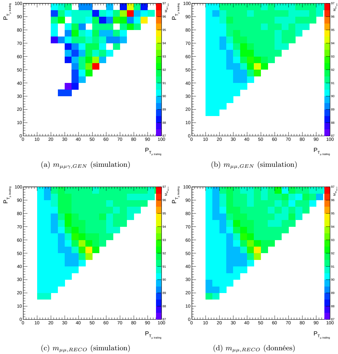
FIGURE 4.17 – Validité de la correspondance m_{\mu\mu\gamma, GEN} \rightarrow m_{\mu\mu, GEN} \rightarrow m_{\mu\mu, RECO} dans la simulation (resp. 4.17a, 4.17b et 4.17c) et comparaison entre simulation (figure 4.17c) et données (figure 4.17d). Les corrections à l'échelle d'impulsion des muons sont appliquées.
