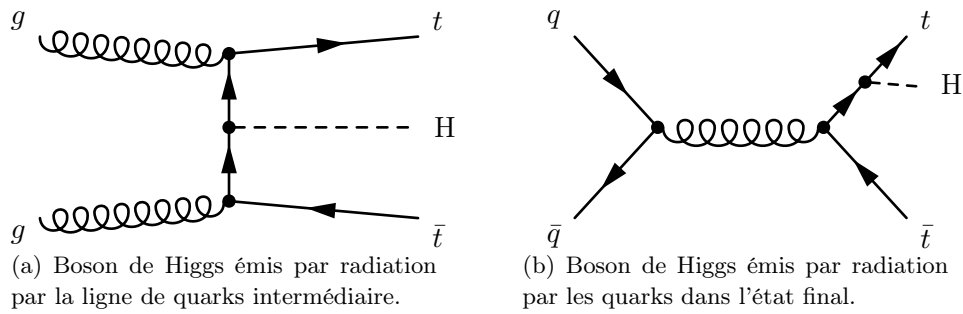
FIGURE 1.10 – Production associée d'un boson de Higgs avec une paire de quarks top.
