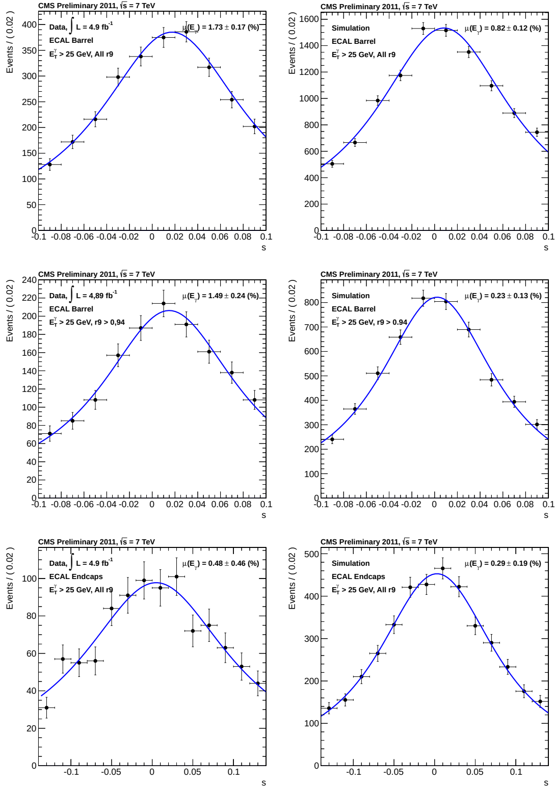
FIGURE 4.24 – Échelle d'énergie des photons s_{RECO} pour les données (gauche) et la simulation (droite), pour les photons sélectionnés d'énergie transverse E_T^\gamma > 25 \text{ GeV} . Les photons sont détectés dans le tonneau (haut), dans le tonneau avec R_9 > 0.94 (milieu) ou dans les bouchons (bas). Les données sont reconstruites avec la calibration du 16 janvier. Les données et la simulation utilisent la régression pour la correction en énergie des photons et les corrections Rochester pour l'impulsion des muons. Ces résultats ont été rendus publics dans [86].
