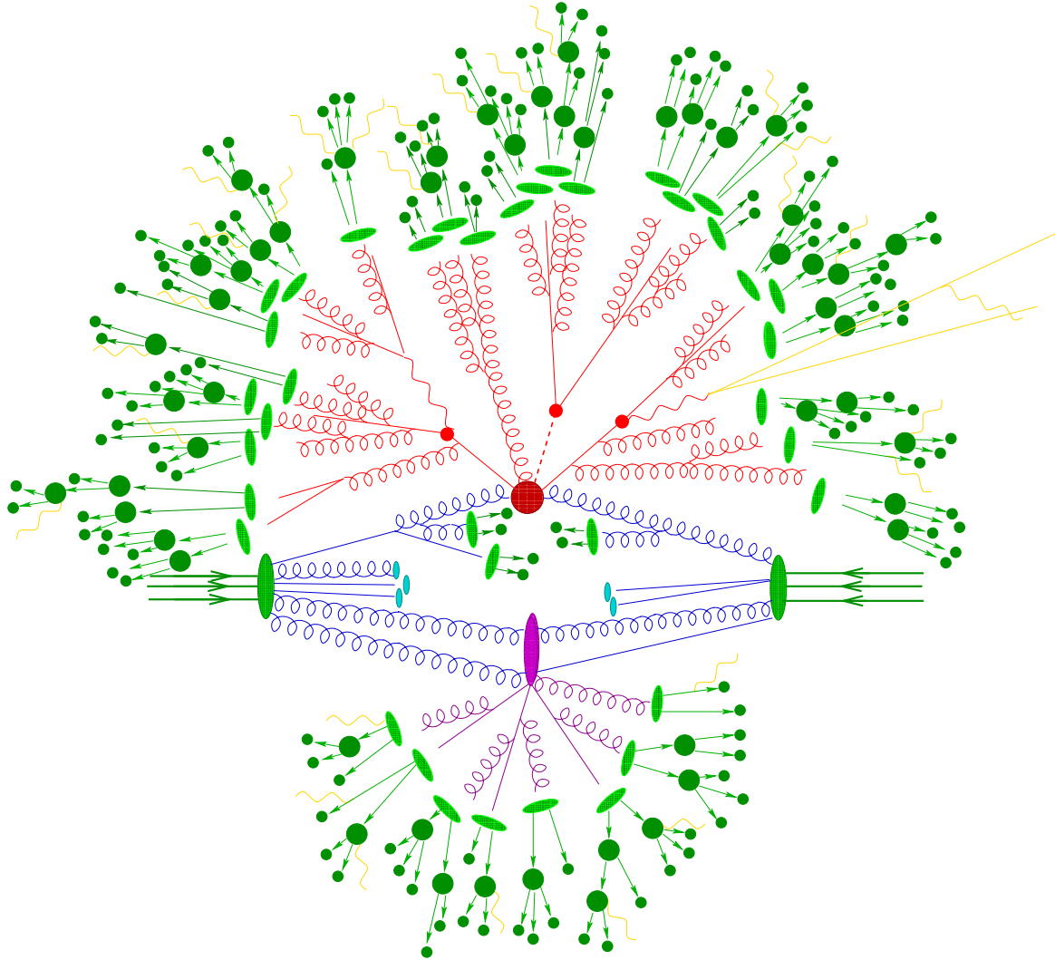
FIGURE 2.21 – Représentation schématique d'un événement t\bar{t}h produit par un générateur d'événements. L'interaction dure (vertex rouge foncé) est suivie par la désintégration des deux quarks tops et du boson de Higgs (vertex rouge clair). De la radiation QCD dure est produite (rouge) et une interaction secondaire peut avoir lieu (vertex violet). Les partons dans l'état final sont ensuite hadronisés (vertex vert clair), et les hadrons se désintègrent (vertex vert foncé). La radiation de photon (jaune) peut avoir lieu à n'importe quelle étape. Les partons à l'état initial n'ayant pas interagi (vertex bleu clair) sont également hadronisés : il s'agit de l'événement sous-jacent. Figure tirée de [54].
