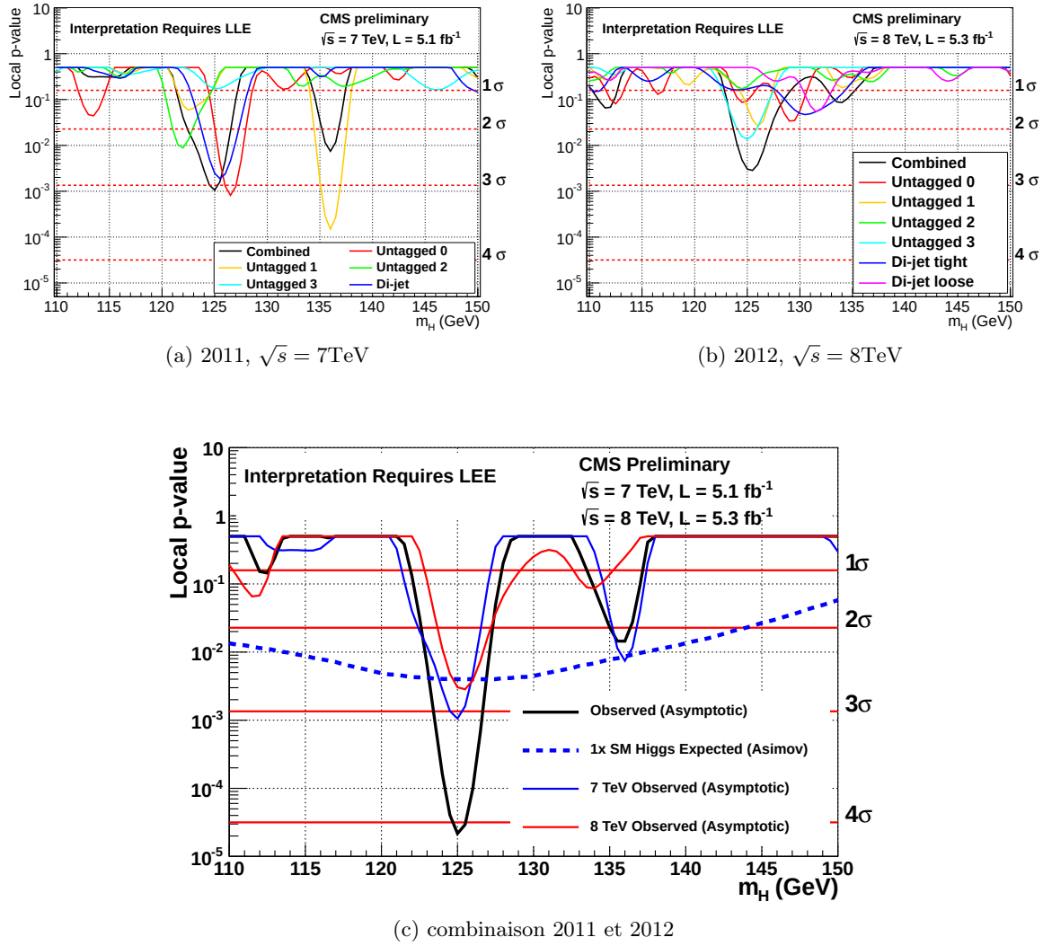
FIGURE 5.27 – p -value locale observée en fonction de l'hypothèse de la masse du boson de Higgs m_H dans les données 2011 (a), 2012 (b) et la combinaison des données 2011 et 2012 (c). Tiré de [92].
