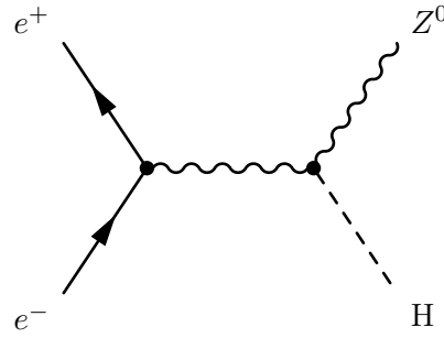
FIGURE 1.18 – Production d'un boson de Higgs par Higgsstrahlung en collisions e^+e^- .
