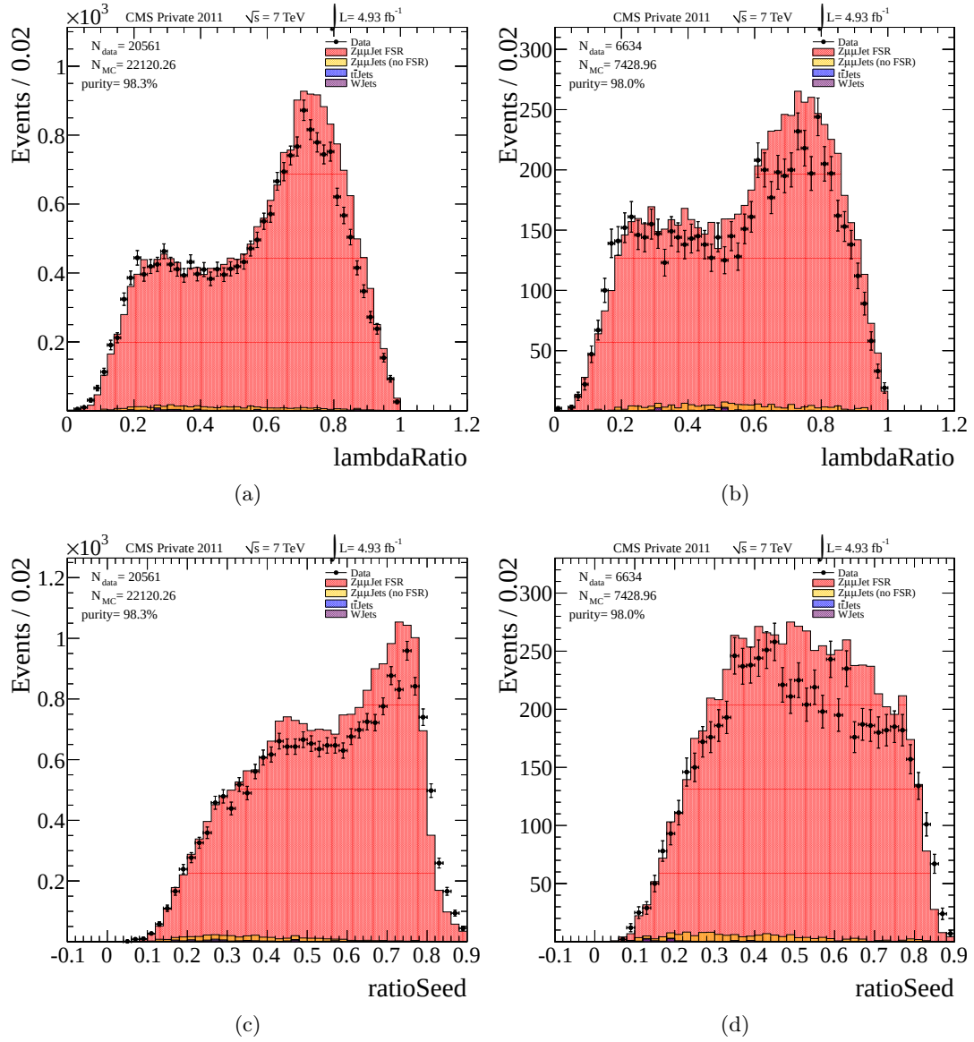
FIGURE A.1 – Comparaisons données-simulation pour les données 2011 avec la calibration du 16 janvier.
