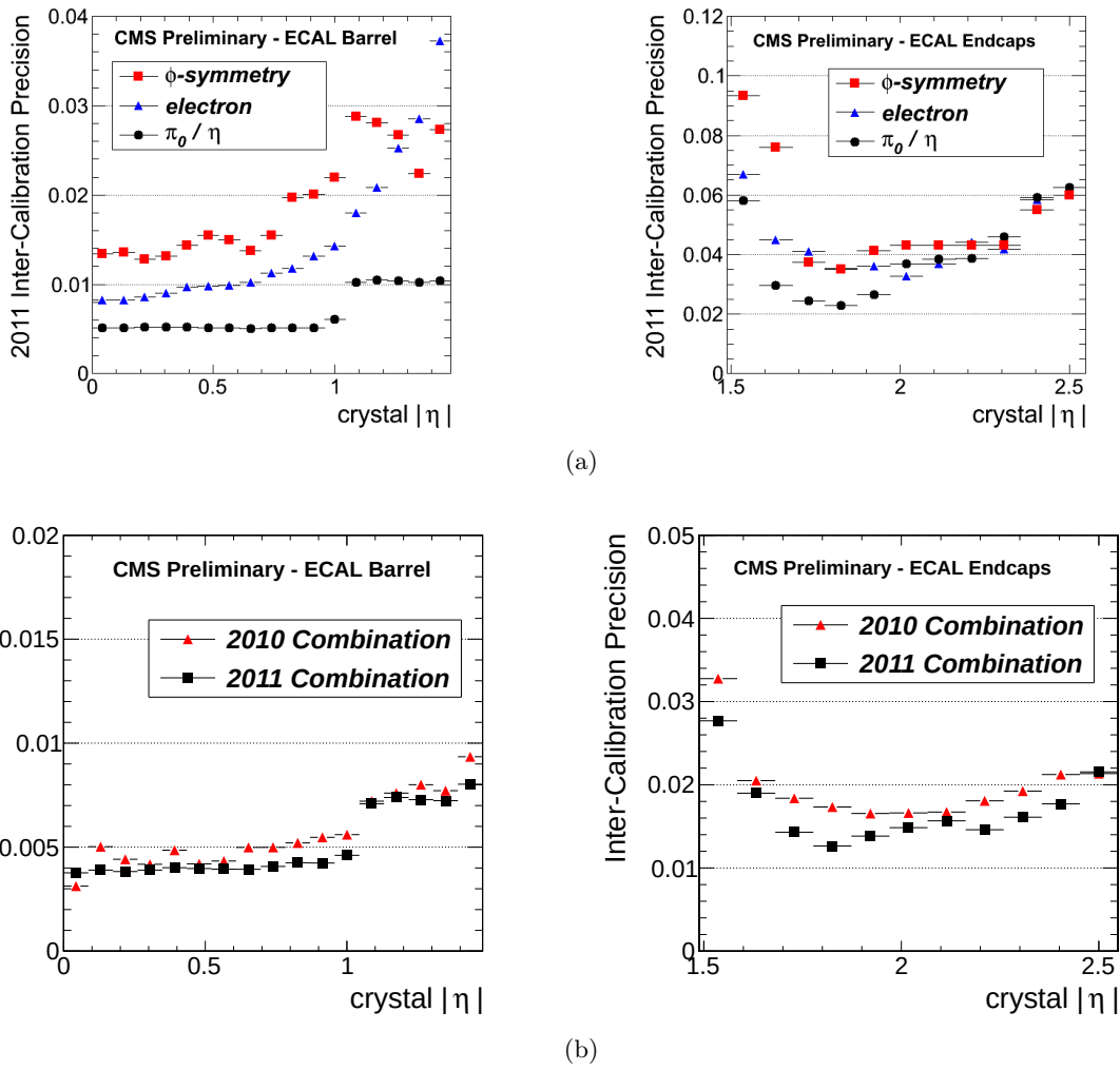
FIGURE 3.20 – Précision des différentes méthodes d'inter-calibration (haut, tiré de [68]) et précision de la combinaison de ces méthodes (bas, tiré de [67]), pour le tonneau (gauche) et les bouchons (droite).
