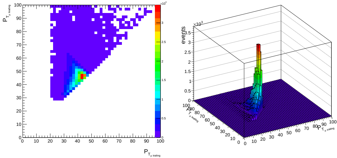
FIGURE 4.16 – Densité d'événements FSR dans le plan (p_T^{lead}, p_T^{trail}) dans la simulation.
