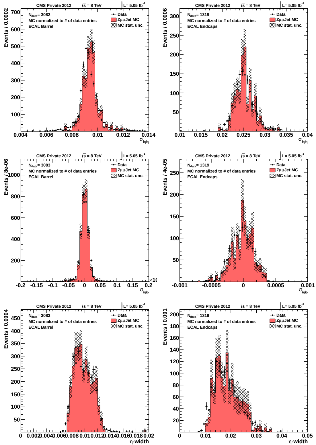
FIGURE 5.6 – Distributions des variables de forme du cluster \sigma_{i\eta i\eta} (haut), \sigma_{i\eta i\phi} (milieu) et \sigma_\eta (bas) pour le tonneau (gauche) et les bouchons (droite) dans les événements Z^0 \rightarrow \mu\mu\gamma .
