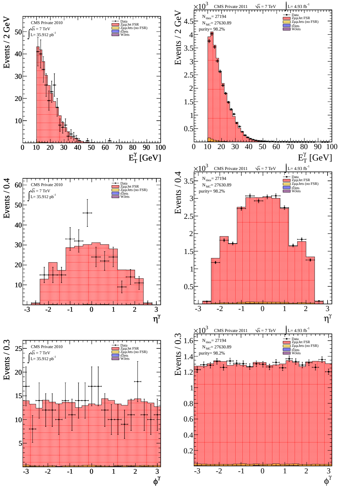
FIGURE 4.5 – Comparaisons données simulation pour les données 2010 (gauche) et les données 2011 avec la calibration du 16 janvier (droite), illustrant quelques variables cinématiques du photon provenant de la radiation dans l'état final : énergie transverse E_T^\gamma (haut), pseudo-rapidité \eta^\gamma (milieu) et azimut \phi^\gamma (bas).
