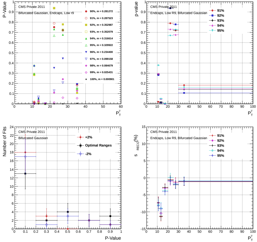
FIGURE 4.29 – Figures de mérite de la stabilité de l’ajustement pour s_{RECO} , pour la catégorie des boudons à bas R_9 . La figure en haut à gauche présente la p -value de l’ajustement pour différentes plages d’ajustement en fonction de l’impulsion transverse du photon. La figure en haut à droite présente la p -value de l’ajustement en fonction de l’impulsion transverse du photon pour la plage d’ajustement choisie à plus ou moins 2 %. La figure en bas à gauche présente l’histogramme du nombre d’ajustements, toutes catégories superposées, en fonction de la p -value. La figure en bas à droite présente les valeurs de l’échelle d’énergie ajustées en fonction de l’impulsion transverse du photon, pour la plage d’ajustement choisie à plus ou moins 2 %.
