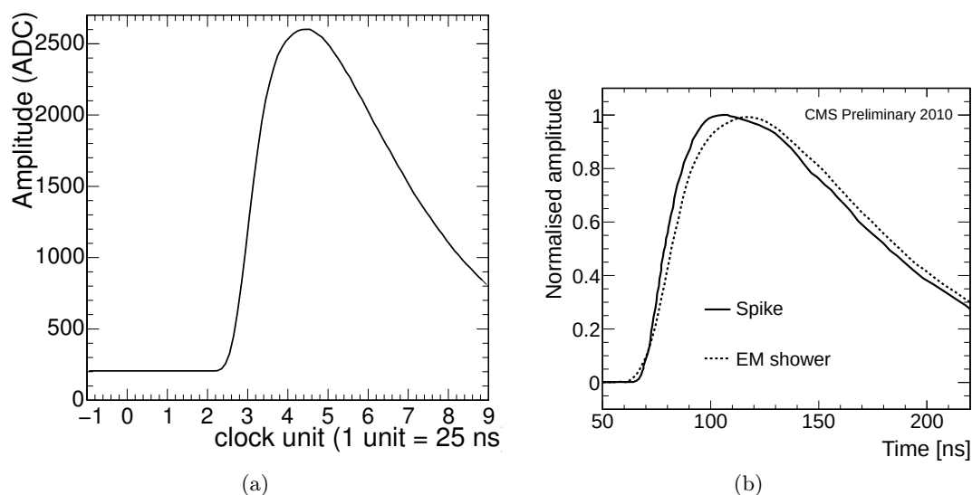
FIGURE 3.9 – Forme du pulse d’une gerbe électromagnétique, pour un électron de 120 GeV (gauche, tirée de [42]), et comparaison entre un pulse normal et un spike (droite, tirée de [63]) : la durée de croissance du pulse est plus marquée que dans le cas d’un signal de lumière de scintillation.
