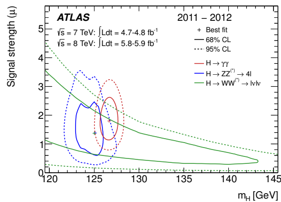
FIGURE C.6 – Ajustement conjoint de la masse du boson de Higgs m_H et de sa section efficace \mu = \sigma/\sigma_{SM} dans l'expérience ATLAS : contours à 68 % (pointillés) et 95 % (trait plein) du niveau de confiance séparé pour les différents canaux étudiés. La croix indique la valeur du meilleur ajustement. Figures tirées de [107].
