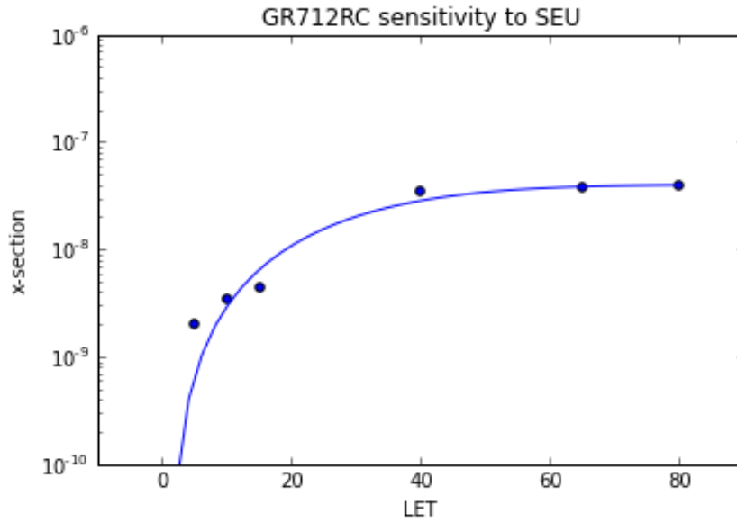
Figure 71 GR712RC bit SEU cross-section
