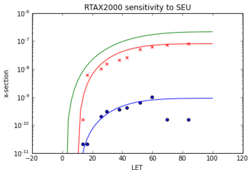
Figure 72 RTAX2000 R-cells SEU cross-sections
