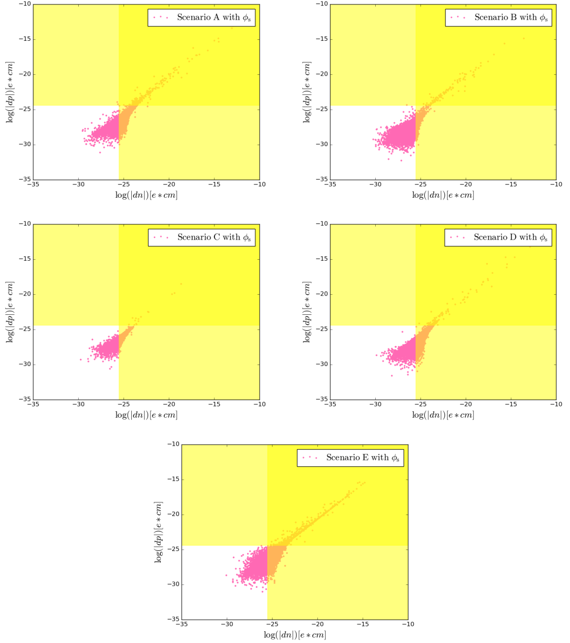
Figure 9.10: EDM del neutrón vs EDM del neutrón para los escenarios A (parte superior izquierda), B (parte superior derecha), C (parte intermedia izquierda), D (parte intermedia derecha) y E (parte inferior). La parte sombreada amarilla se corresponde con la región excluida por el actual límite en los EDM del neutrón [256] y del mercurio [252].
