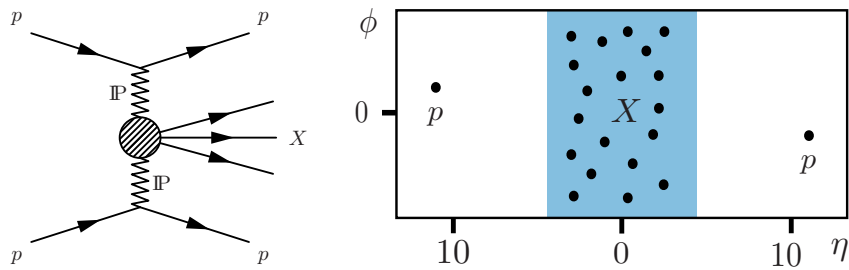
(d) Central diffraction (CD)
