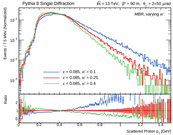
(d) MBR – varying \alpha' , keeping \epsilon constant.
