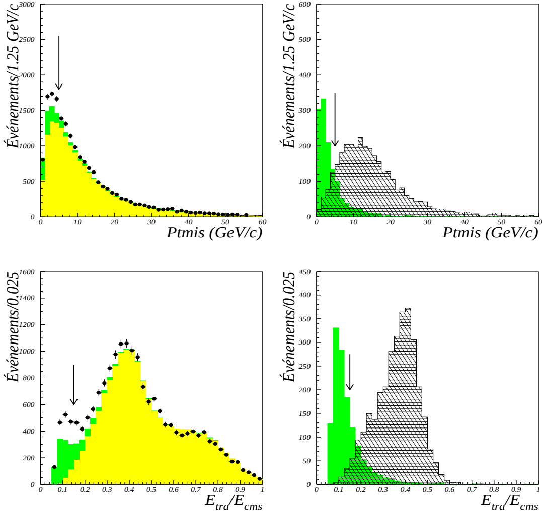
Figure 5.2: Les figures de gauche montrent les distributions de P_{t\text{mis}} et E_{\text{tra}}/E_{\text{cms}} obtenues dans les données et celles prédites à partir de la simulation pour les processus standards. La normalisation est fixée par la luminosité enregistrée et par les valeurs des sections efficaces prédites pour les différents processus. Les figures de droite correspondent aux mêmes distributions pour les événements de fond \gamma\gamma ainsi que pour les événements de signal qui ont été générés à une masse du boson de Higgs de 95 \text{ GeV}/c^2 ; la normalisation du signal est arbitraire. La flèche indique l'endroit où la coupure finale est appliquée.
