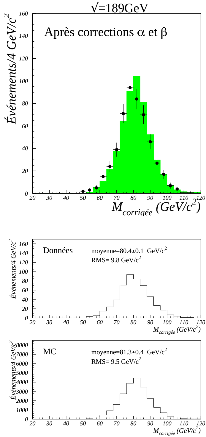
Figure 6.7: Distribution de masse pour les événements W semileptoniques sélectionnés à \sqrt{s} = 189 \text{ GeV} après avoir appliqué les facteurs de correction en fonction de l'énergie et de l'angle des jets.
