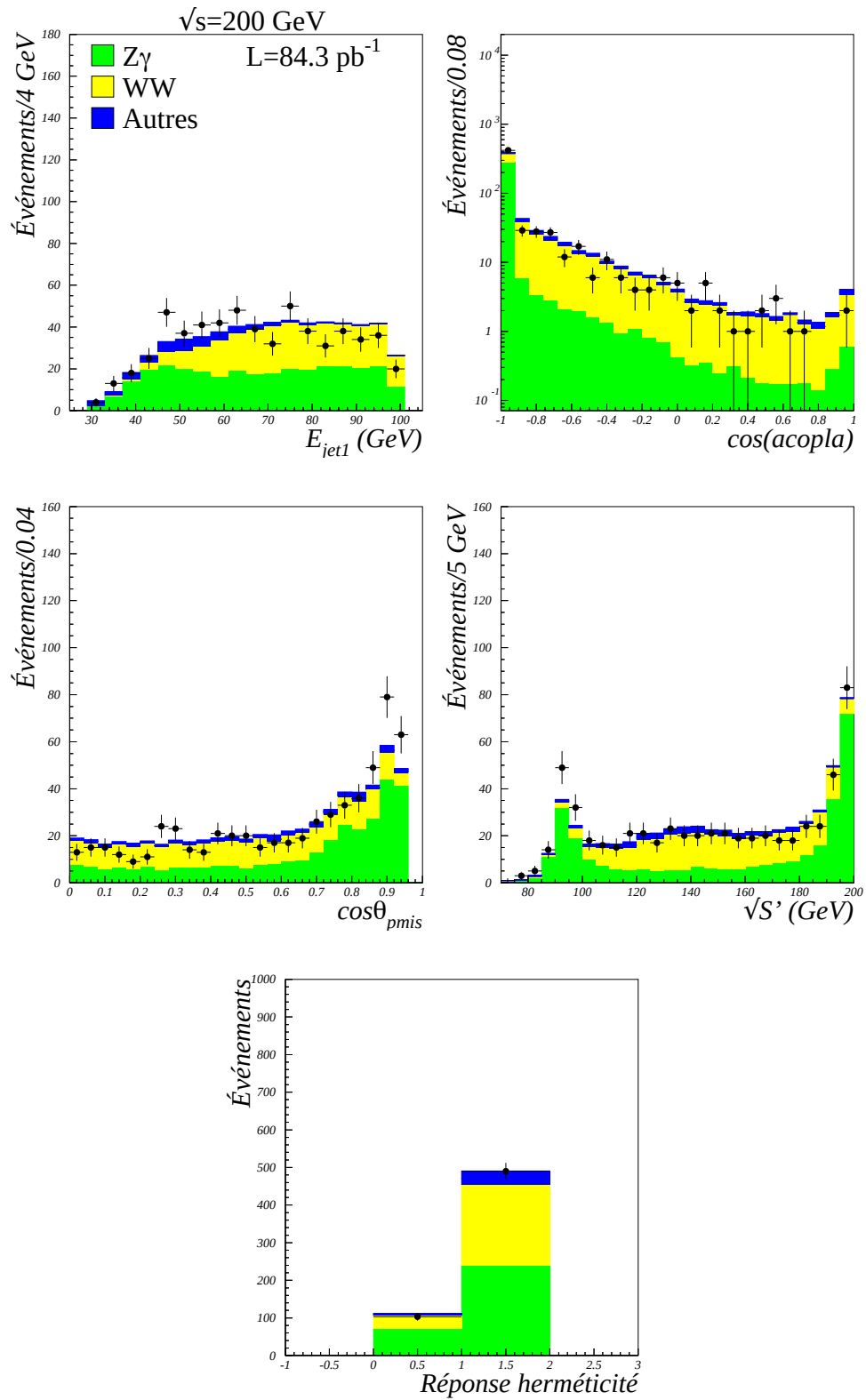
Figure 8.10: Distributions des variables utilisées dans la construction de la variable discriminante pour les 593 événements sélectionnés à \sqrt{s} = 200 GeV. Nous indiquons la contribution de chaque processus standard par différents niveaux de gris.
