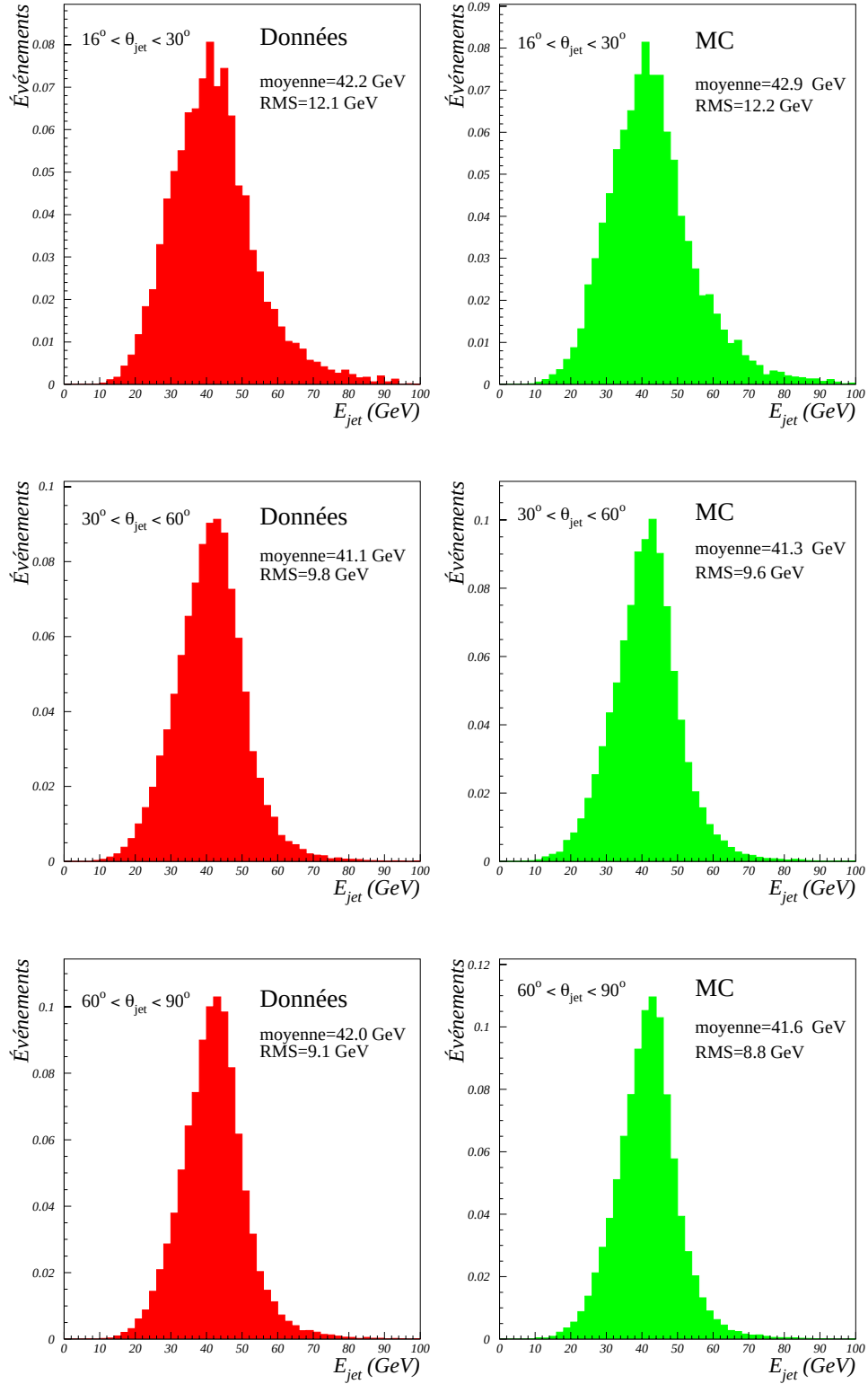
Figure 7.6: Distributions de l'énergie mesurée dans les hémisphères pour les données enregistrées à \sqrt{s} = 91,2 GeV (à gauche) et pour les événements simulés (à droite) en divisant l'échantillon en différentes régions d'angle polaire du jet.
