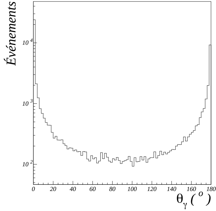
Figure 2.5: En haut, distribution des impulsions axiales( p_z ) des deux photons pour les événements q\bar{q}(n\gamma) générés à \sqrt{s} = 189 \text{ GeV} . En bas, distribution de l'angle polaire généré du photon le plus énergétique reconstruit dans l'événement .
