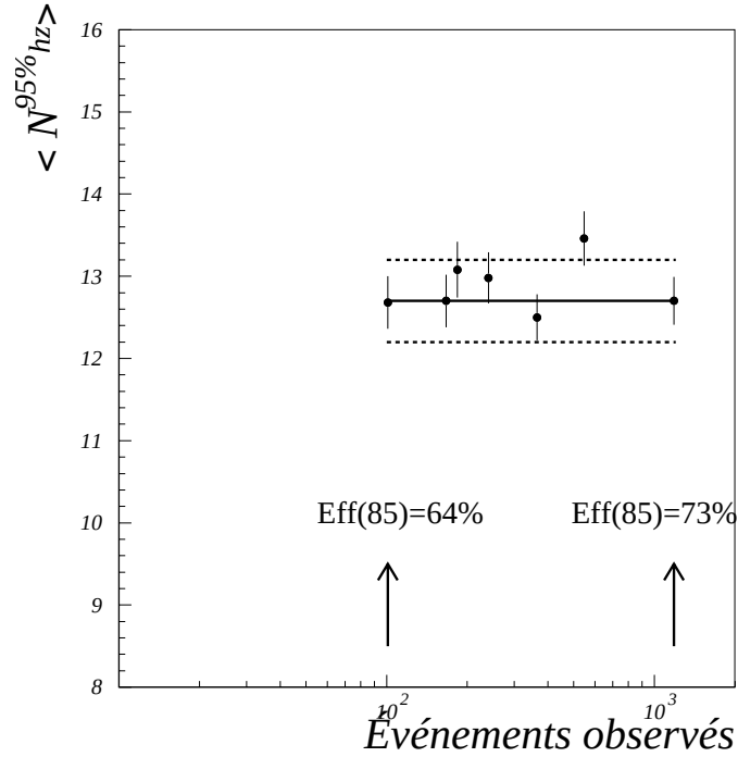
Figure 8.2: Nombre d'événements du signal de boson de Higgs exclus à 95 % de niveau de confiance en fonction du nombre d'événements observés (efficacité). Cet exercice a été fait en utilisant le toy Montecarlo pour une masse générée du boson de Higgs de 85 \text{ GeV}/c^2 . L'efficacité pour le premier point (100 événements observés) est de 64 % et pour le dernier point (1183 événements observés) est de 73,6 %.
