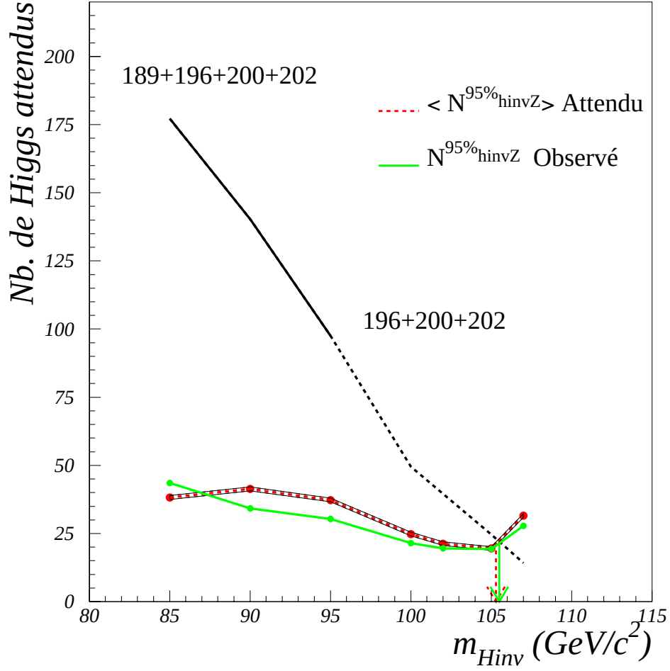
Figure 9.6: Nombre d'événements de signal exclus à 95 % de niveau de confiance en fonction de la masse du boson de Higgs ( \langle N_{h_{inv}Z}^{95\%} \rangle ) pour l'analyse "sliding". La courbe en trait plein qui se continue en trait pointillé donne le nombre d'événements attendus. Pour les points à m_{h_{inv}} = 85, 90 et 95 \text{ GeV}/c^2 nous avons utilisé les données enregistrées à \sqrt{s} = 189, 196, 200 et 202 \text{ GeV} ; pour les masses à partir de m_{h_{inv}} = 100 \text{ GeV}/c^2 nous avons utilisé seulement les données enregistrées à \sqrt{s} = 196, 200 et 202 \text{ GeV} .
