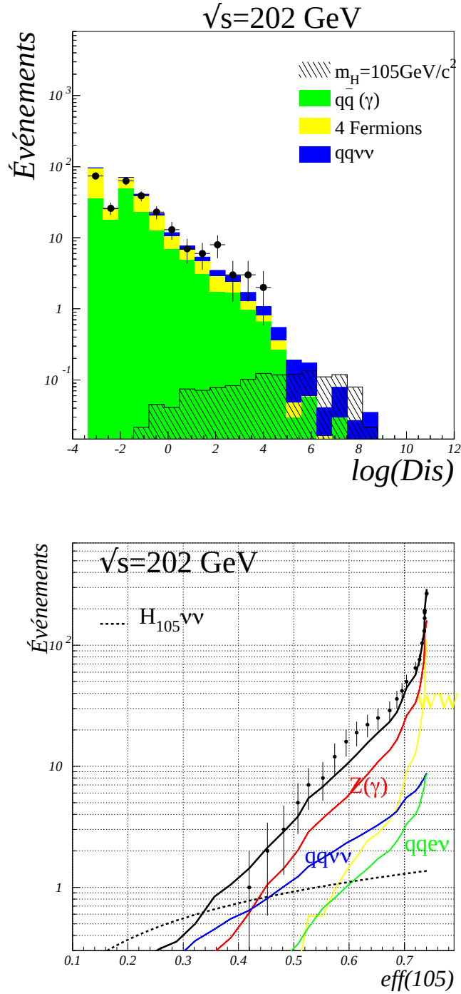
Figure 8.16: Figure du haut: distribution de la variable discriminante ( \log(\text{Dis}) ). Les histogrammes représentent les contributions des différents processus de bruit de fond et les points avec les barres d'erreur indiquent les données réelles. Figure du bas: évolution du nombre d'événements attendus issus des processus standard comparée à celle des données réelles enregistrées à \sqrt{s} = 202 \text{ GeV} en fonction de l'efficacité pour le signal. Les points sont les données réelles, et nous différencions les contributions des bruits de fond dominants (traits pleins) ainsi que le nombre d'événements attendus pour le signal (trait pointillé).
