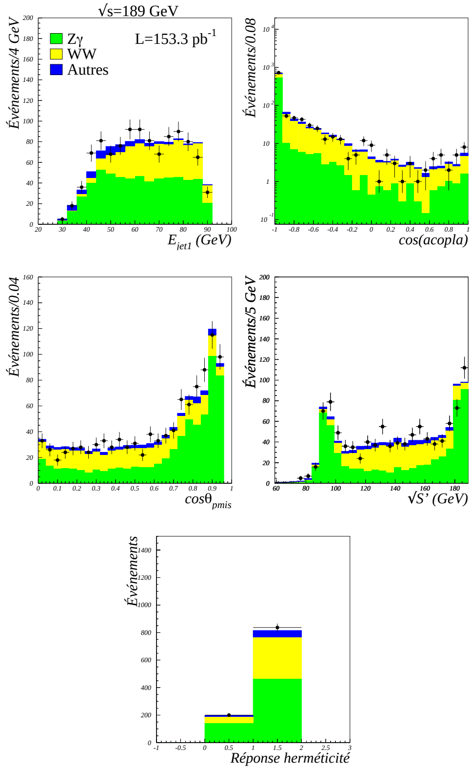
Figure 5.21: Distributions des valeurs des variables utilisées dans la construction de la variable discriminante pour les données enregistrées à \sqrt{s} = 189 \text{ GeV} . Les différentes composantes issues des processus standard sont indiquées.
