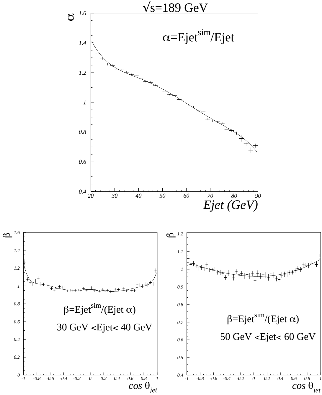
Figure 6.6: En haut, facteur de correction \alpha en fonction de l'énergie du jet. En bas, exemples du facteur de correction \beta en fonction de \cos \theta_{\text{jet}} pour différents bins d'énergie (30–40 et 50–60 GeV). Le facteur \beta est évalué une fois que la correction sur l'énergie a été appliquée ( \alpha E_{\text{jet}} ).
