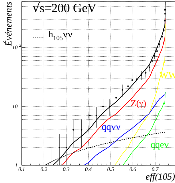
Figure 8.15: Figure du haut: distribution de la variable discriminante ( \log(Dis) ). Les histogrammes représentent les contributions des différents processus de bruit de fond et les points avec les barres d'erreur indiquent les données réelles. Figure du bas: évolution du nombre d'événements attendus issus des processus standard comparée à celle des données réelles enregistrées à \sqrt{s} = 200 GeV en fonction de l'efficacité au signal. Les points sont les données réelles, et nous différencions les contributions des fonds dominants (traits pleins) ainsi que le nombre d'événements attendus pour le signal (trait pointillé).
