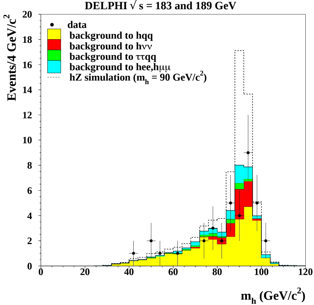
Figure 7.19: Distribution de la masse reconstruite en combinant tous les canaux de recherche du boson de Higgs pour les événements de bruit de fond (histogrammes pleins) et les événements réels (points). La contribution des différents canaux est indiquée. La distribution attendue pour le signal généré avec une masse de 90 \text{ GeV}/c^2 a été additionnée à la distribution des événements de bruit de fond.
