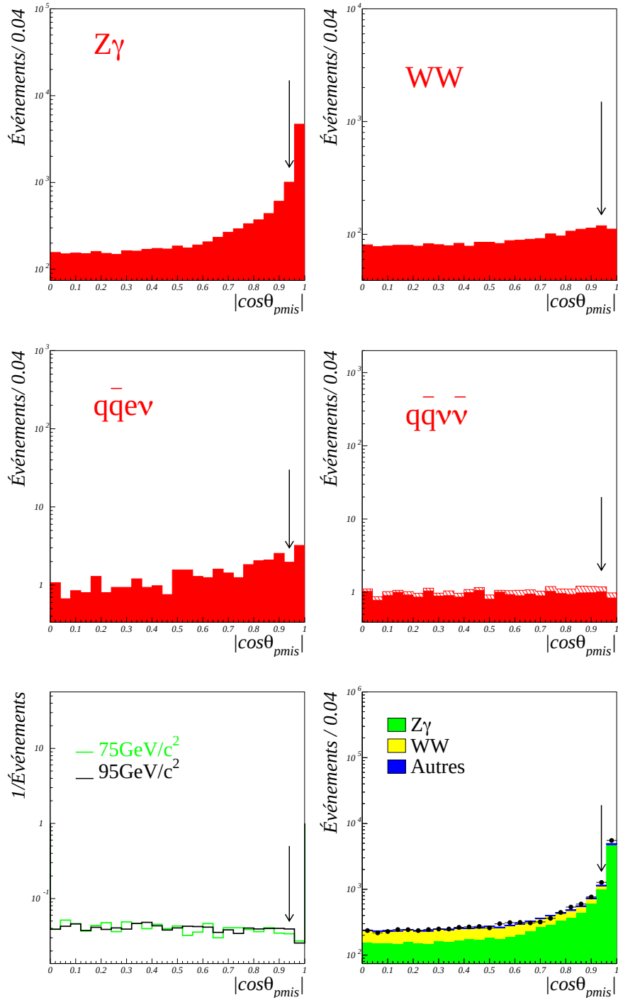
Figure 5.7: Distributions du cosinus de l'angle \theta_{pmis} de l'impulsion manquante pour les fonds principaux normalisées à la luminosité enregistrée, pour les données et pour les événements de signal qui ont été générés avec une masse de boson de Higgs de 75\text{ GeV}/c^2 et 95\text{ GeV}/c^2 . Les distributions des événements de signal sont normalisées à l'unité. Dans la distribution correspondant au processus q\bar{q}\nu\bar{\nu} on a distingué la contribution “ZZ” où les deux bosons sont sur leur couche de masse (histogramme plein) et celle “Z \gamma^* ” avec un boson hors couche de masse (histogramme hachuré). La flèche indique l'endroit où la coupure est appliquée.
