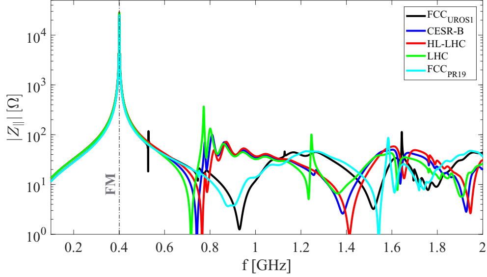
(a) Longitudinal impedance
