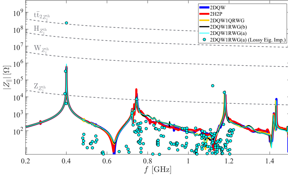
(a) Longitudinal impedance
