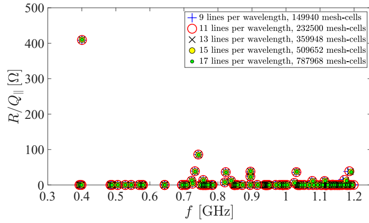
(b) Longitudinal shunt impedance
