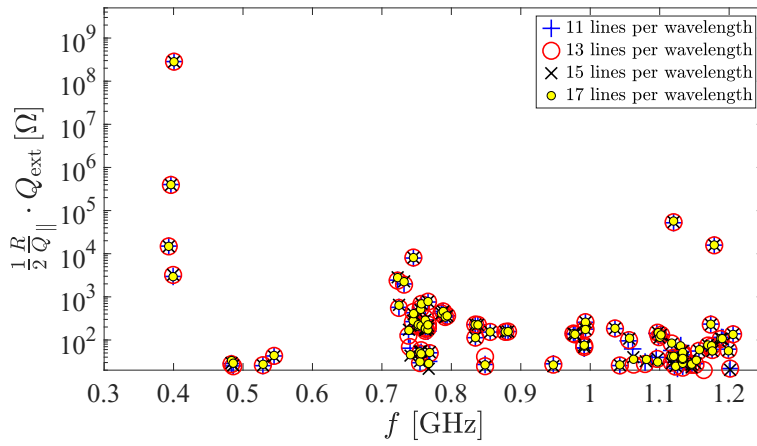
(b) Longitudinal impedance
