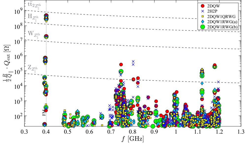
(a) Longitudinal impedance
