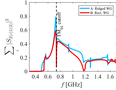
(d) Coupling of the TM_{01} mode of P1 to P2
